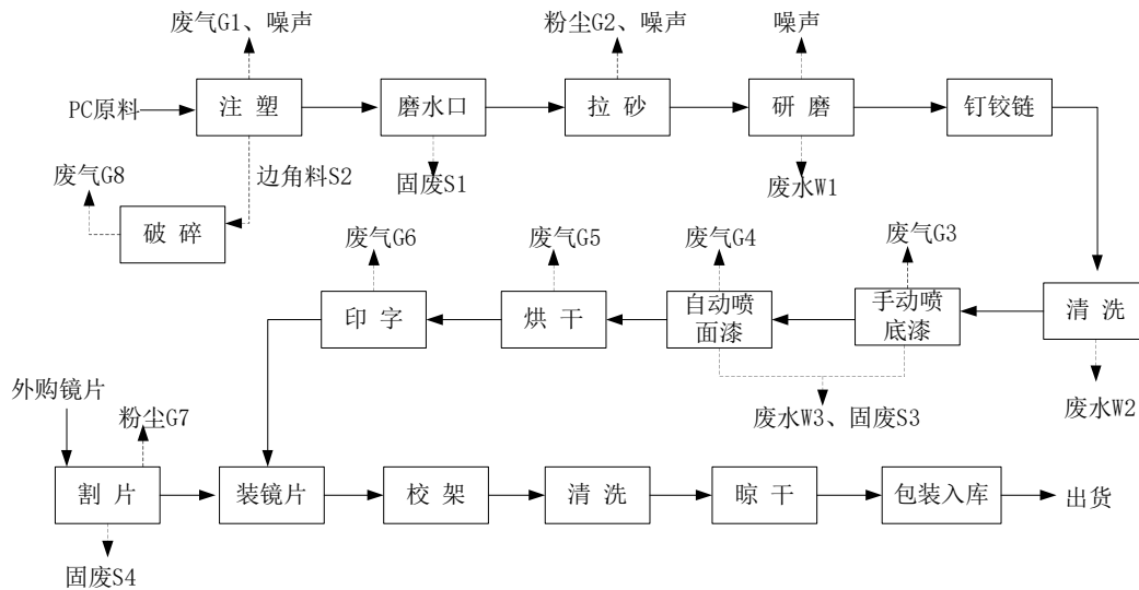
图 3.1-1 原有项目塑料眼镜生产工艺流程图
