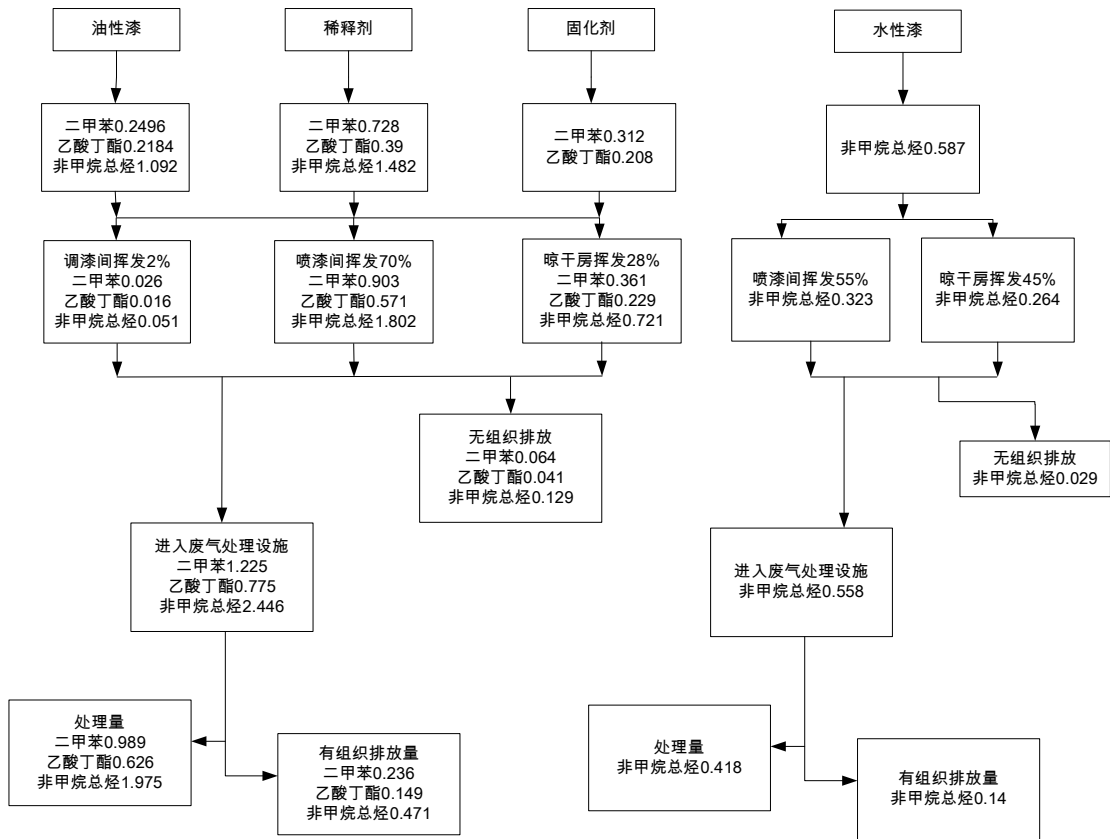
图 4.3-1 项目油漆有机溶剂用量平衡图 单位 t/a
