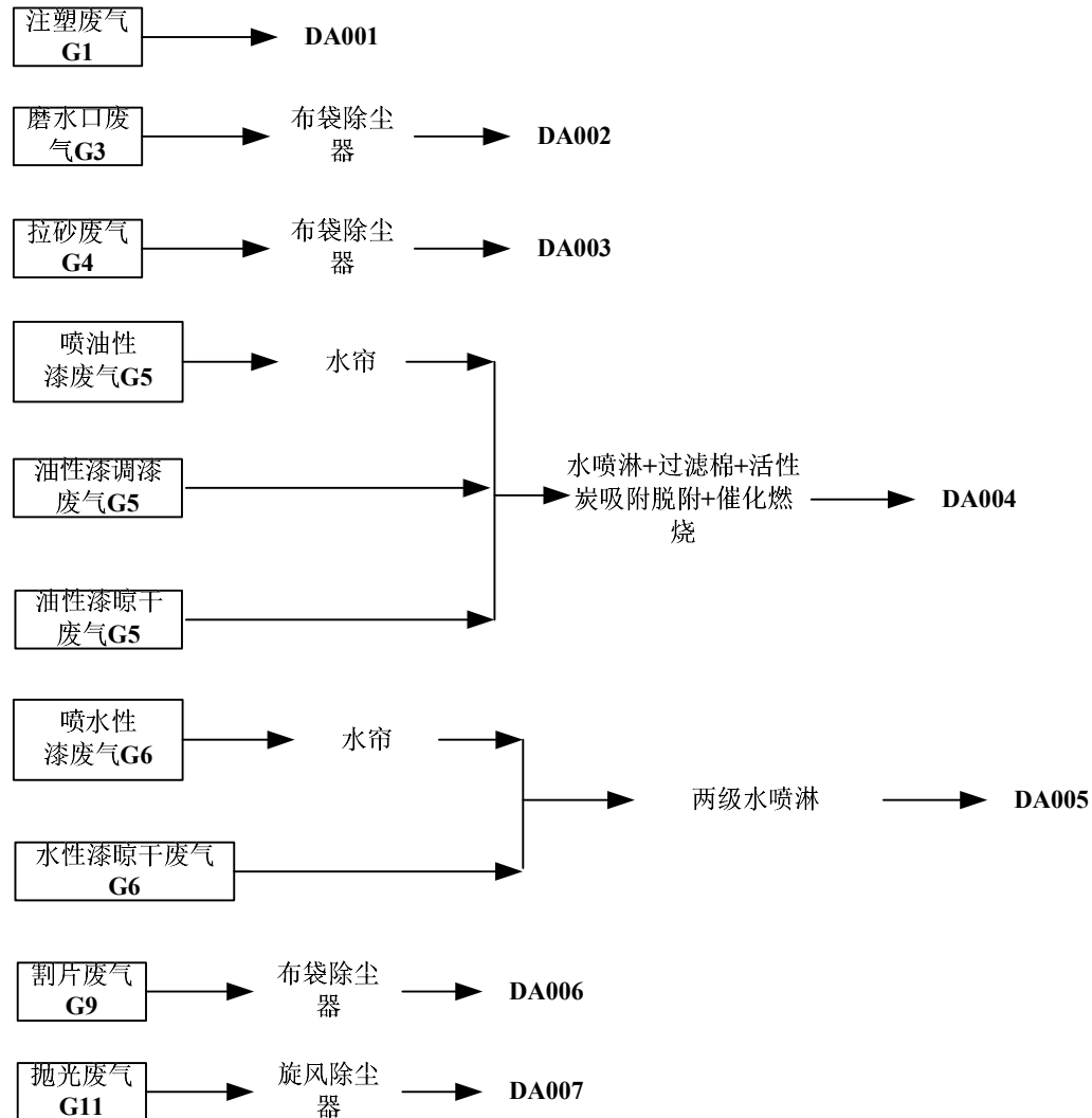
图 7.1-1 项目废气处理工艺流程图
