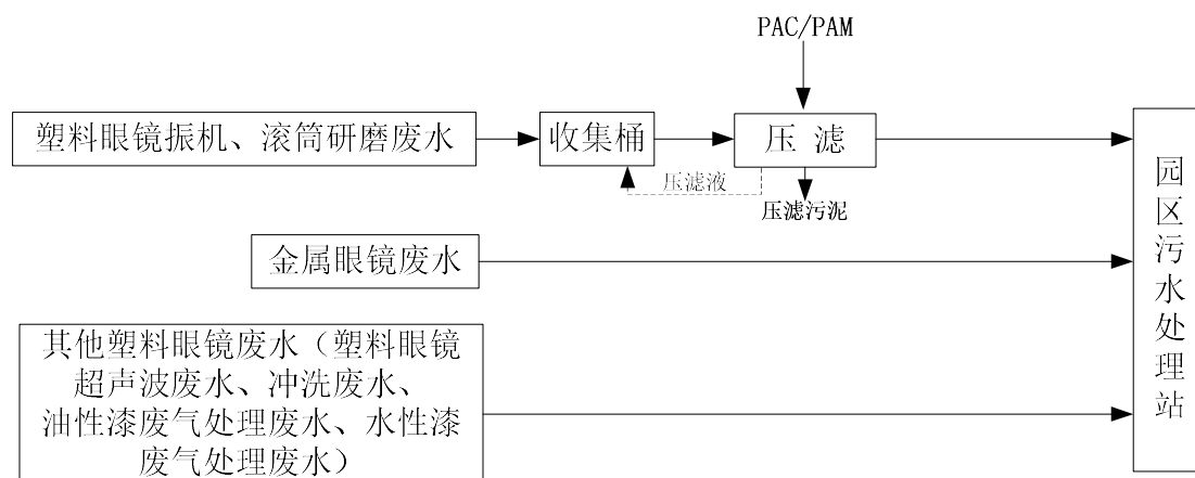
图 7.1-3 企业污水处理工艺图
