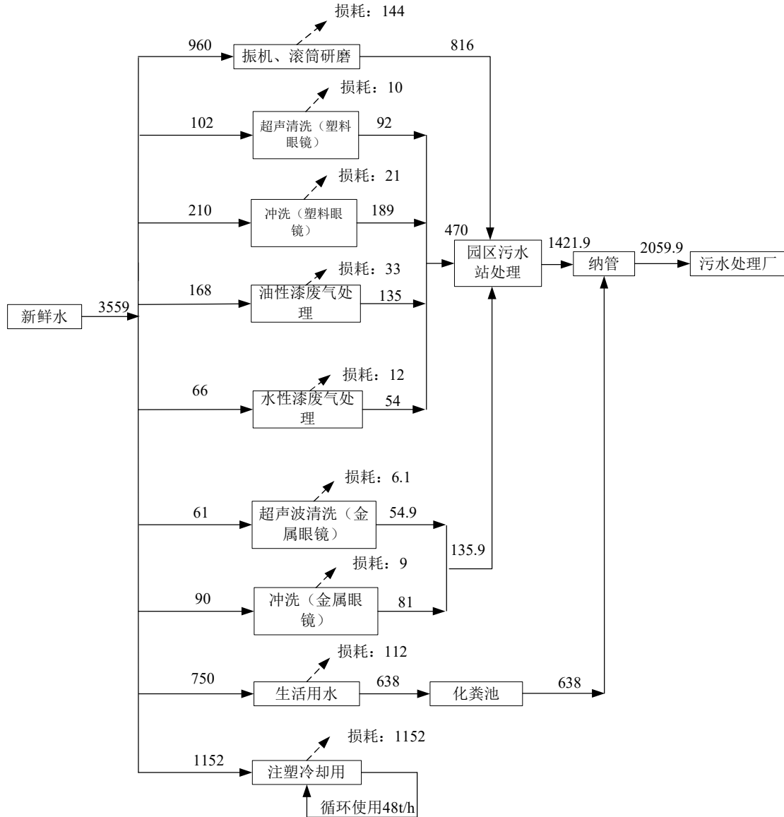
图 4.3-4 项目水平衡图 单位:t/a
