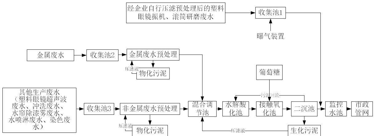
图 7.1-4 杜桥眼镜创业园区污水处理站处理工艺流程图
