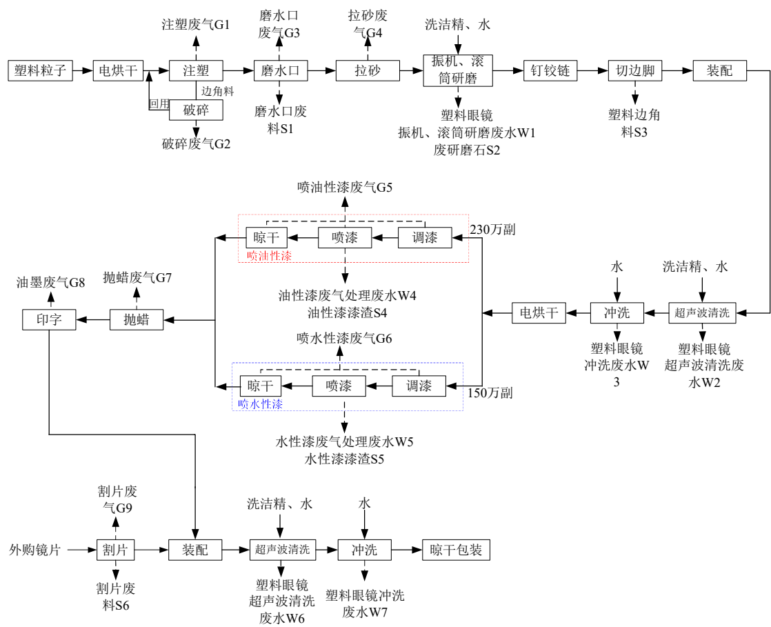
图 4.2-1 项目塑料眼镜生产工艺流程图
