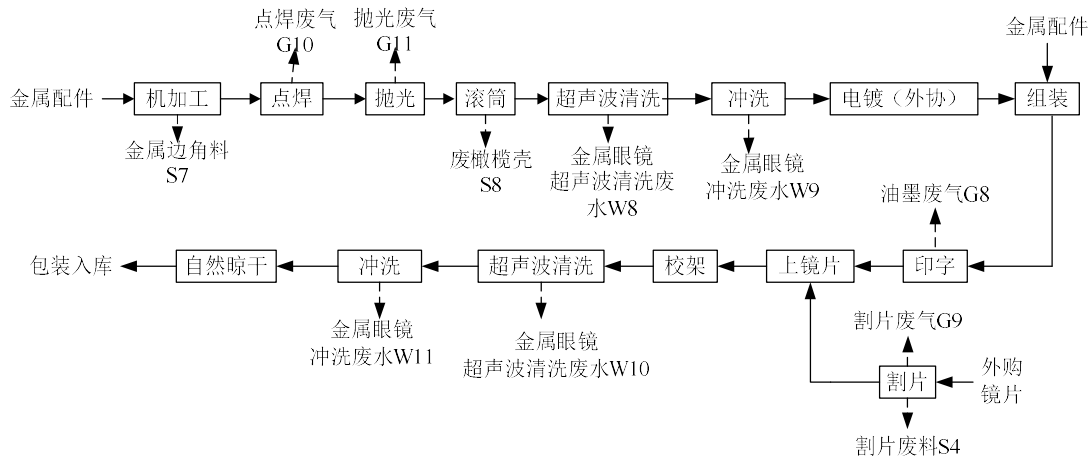
图 4.2-2 项目金属眼镜生产工艺流程图
