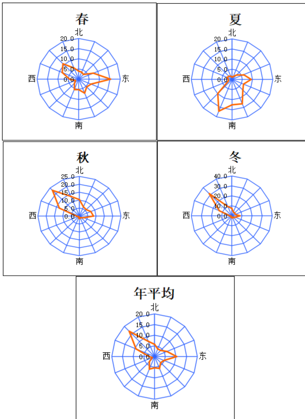
图 6.1-4 风向玫瑰图
