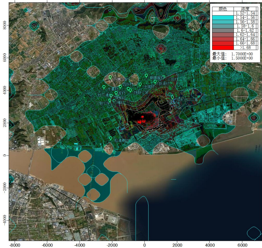
图 6.1-9 非甲烷总烃叠加本底后小时平均浓度分布图 ( \text{mg}/\text{m}^3 )
