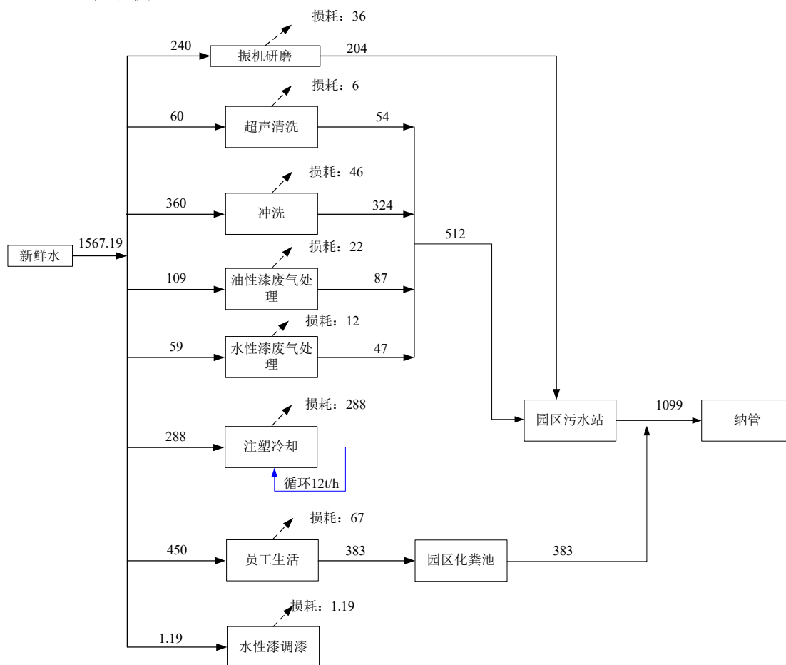
图 3.3-2 项目水平衡图 单位:t/a
