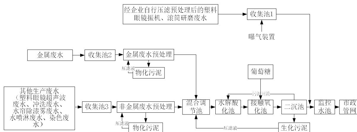
图 6.1-4 杜桥眼镜创业园污水处理站处理工艺流程图
