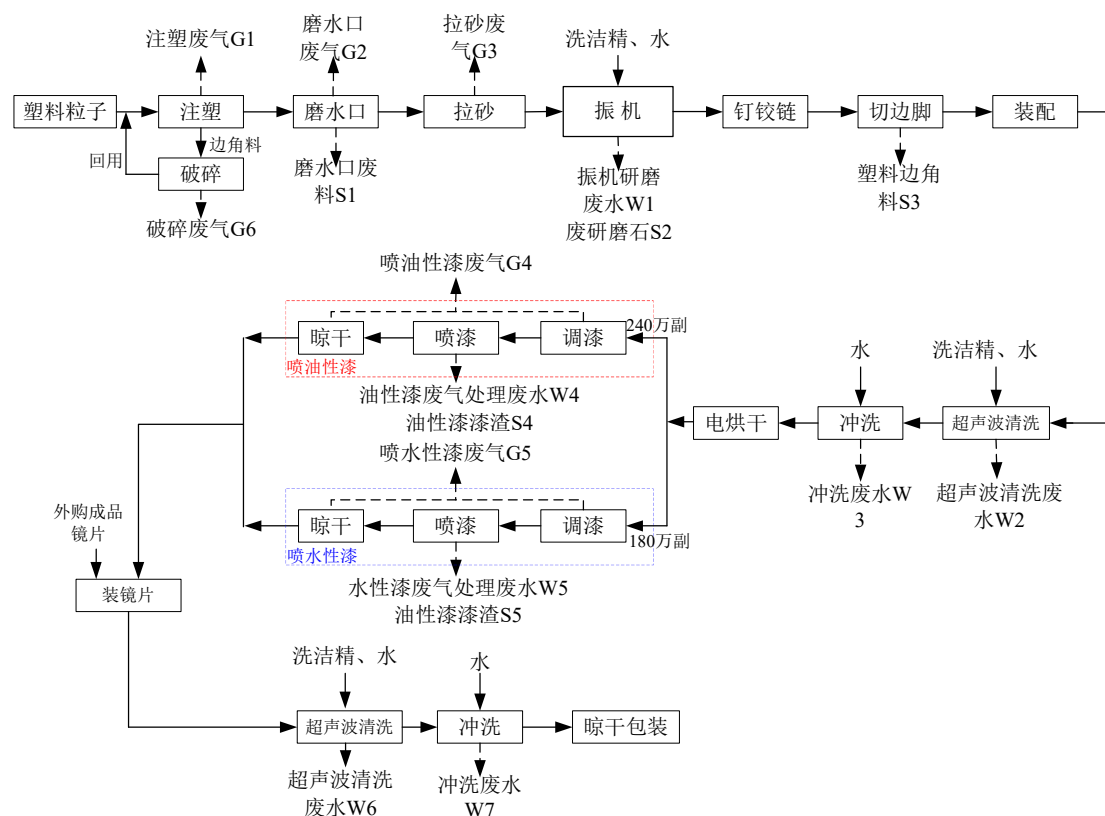
图 3.2-1 项目塑料眼镜生产工艺流程图
