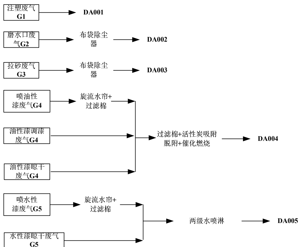
图 6.1-1 项目废气处理工艺流程图
