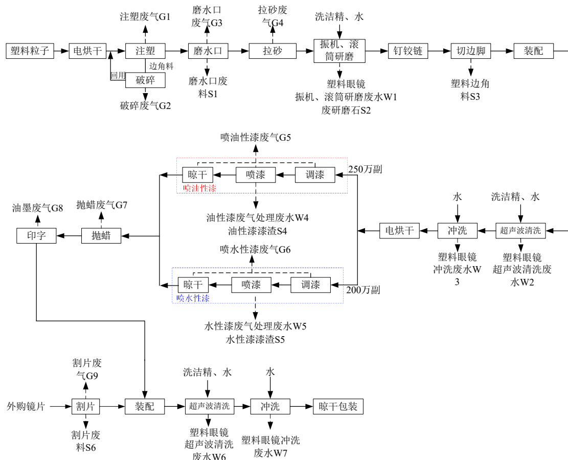
图 3.2-1 项目塑料眼镜生产工艺流程图
