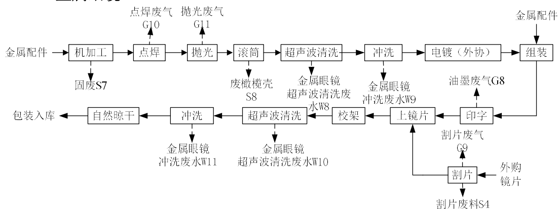
图 3.2-2 项目金属眼镜生产工艺流程图
