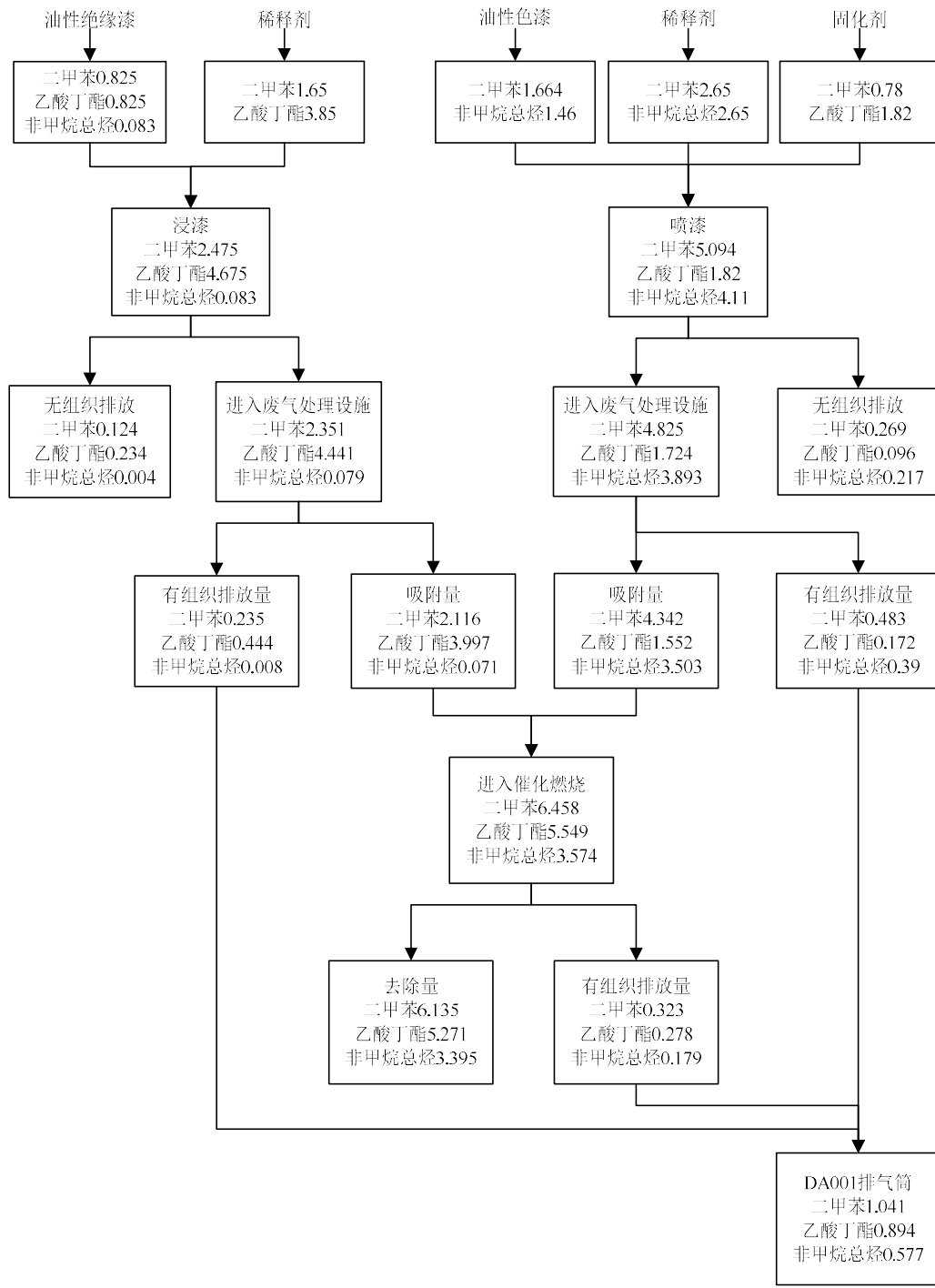
图 3.3-1 油性漆浸漆、喷漆工段有机溶剂平衡图单位: t/a
