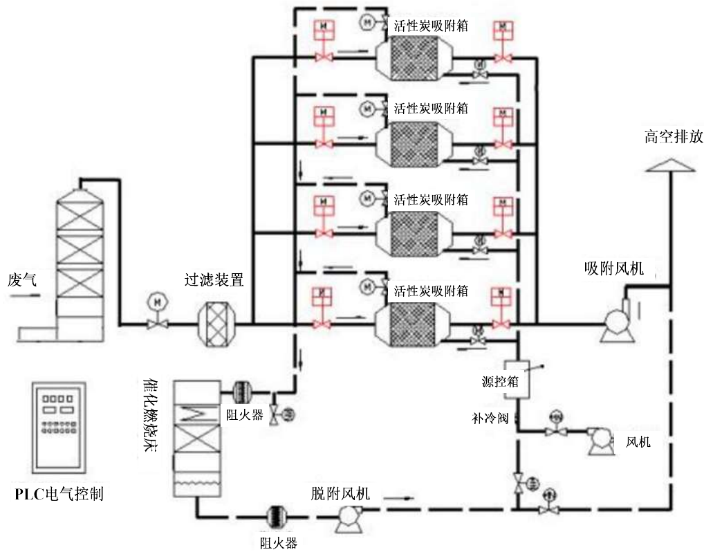
图 6.1-2 处理工艺
