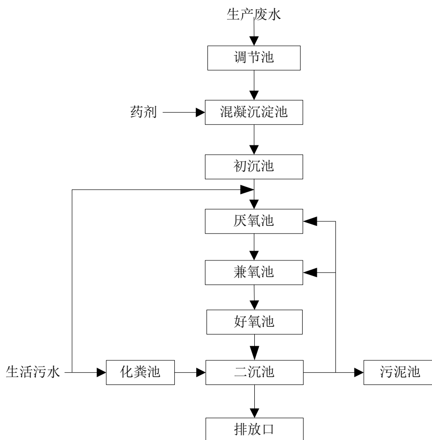
图 6.1-1 建议的污水处理工艺流程图
