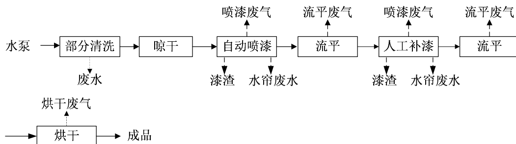
图 3.2-1 油性漆喷漆流水线工艺流程图
