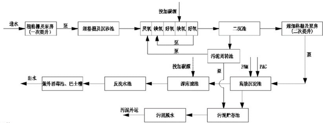
图 2.7-2 二期污水处理工艺流程图
