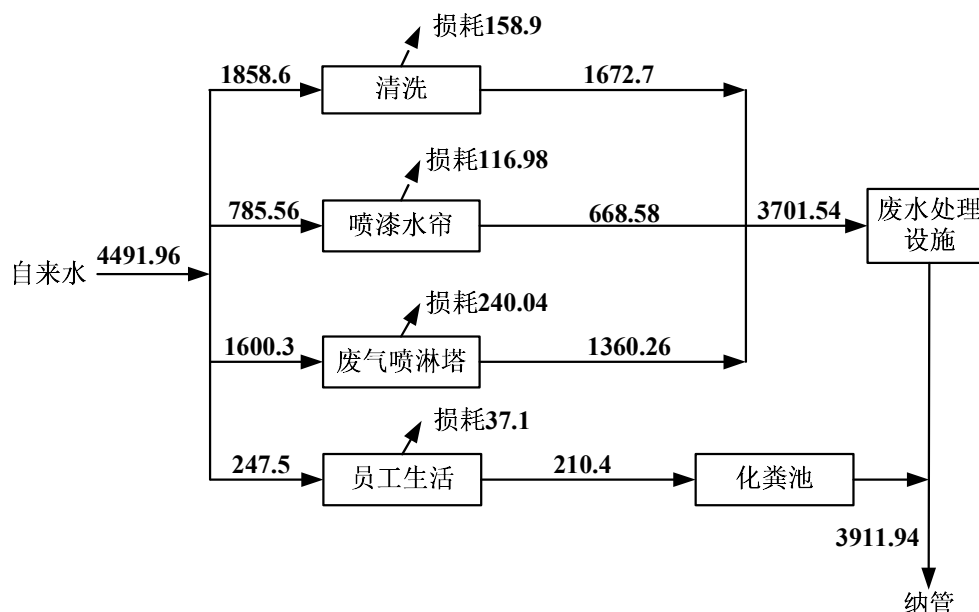
图 3.3-3 项目水平衡图单位：t/a
