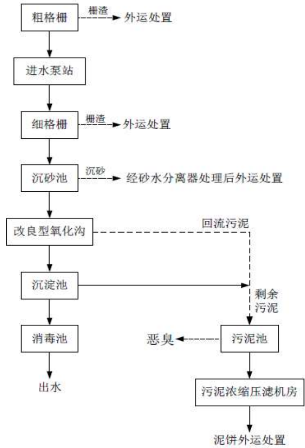
图 2.7-1 一期污水处理工艺流程图
