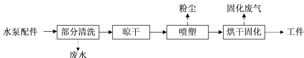
图 3.2-5 水泵配件喷塑工艺流程图
