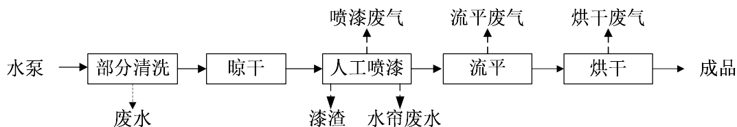
图 3.2-2 水性漆喷漆流水线工艺流程图
