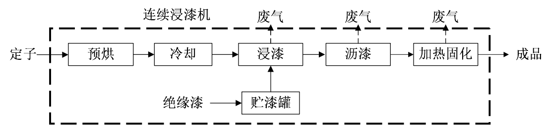
图 3.2-4 定子浸漆工艺流程图
