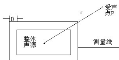
图 5.2-1 Stueber 模型
