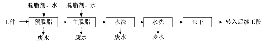
图 3.2-3 清洗工艺流程图
