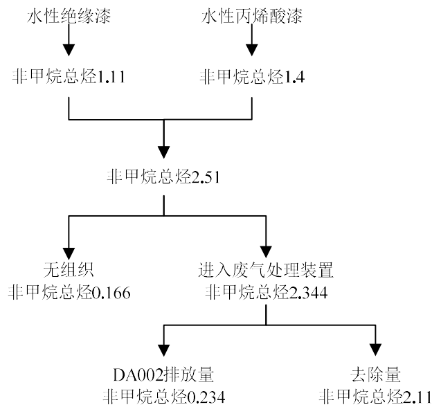
图 3.3-2 水性漆浸漆、喷漆工段有机溶剂平衡图单位：t/a
