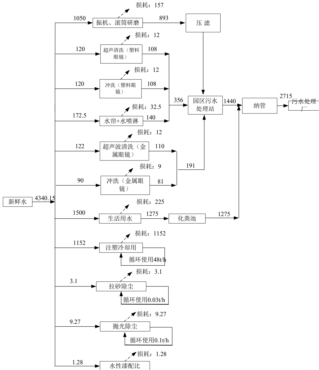
图 3.3-4 项目水平衡图 单位:t/a
