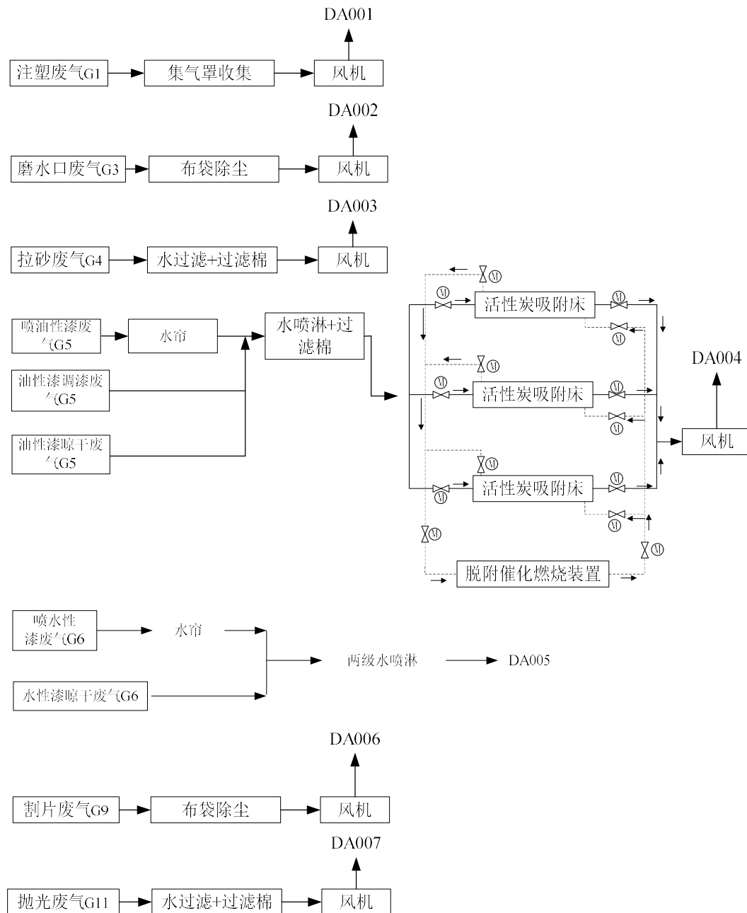
图 6.1-1 项目废气处理工艺流程图
