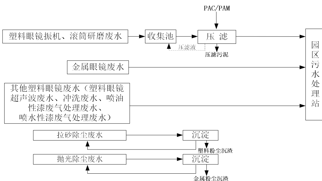
图 6.1-3 企业污水处理工艺图
