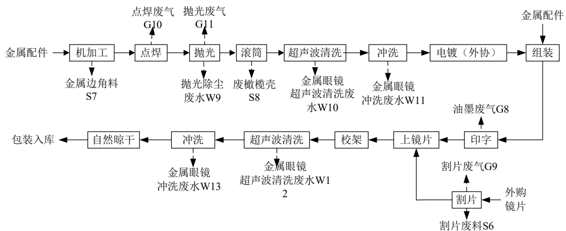
图 3.2-2 项目金属眼镜生产工艺流程图
