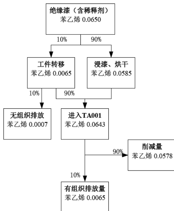
图2-2 绝缘漆溶剂平衡图 (t/a)
