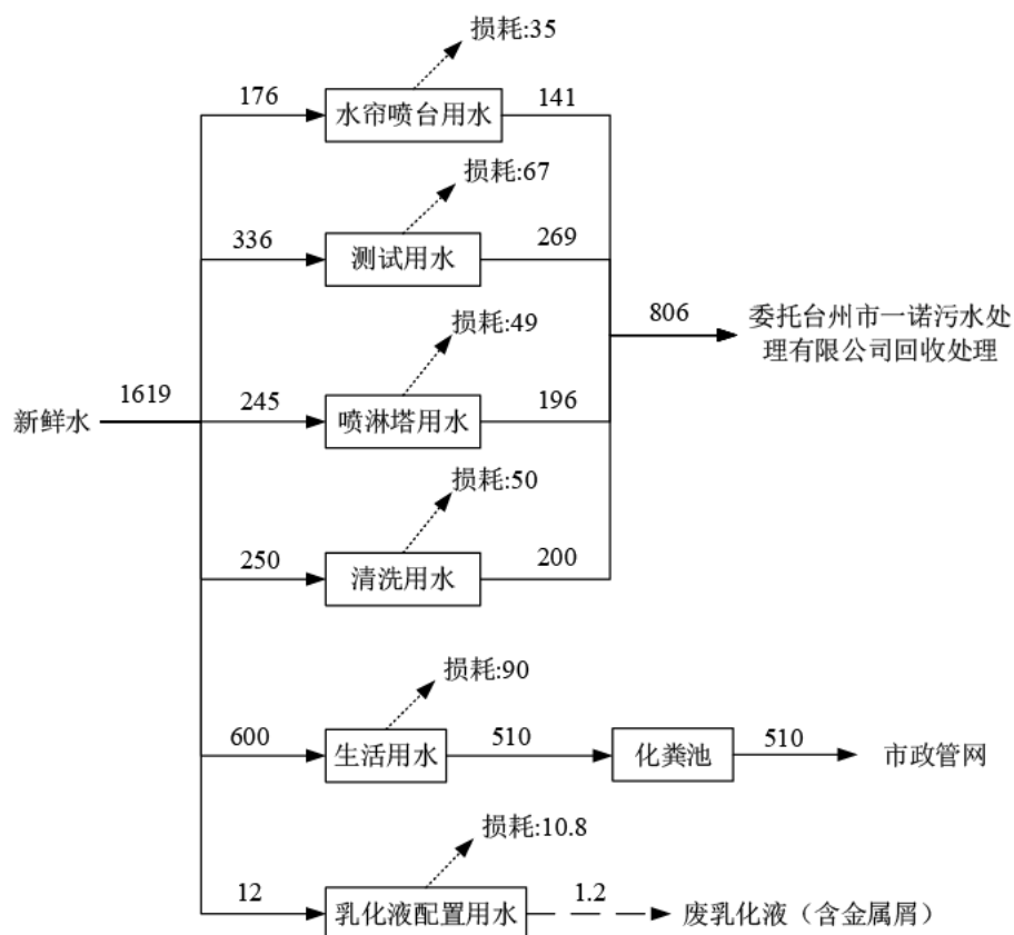
图2-3 水平衡图 (t/a)
