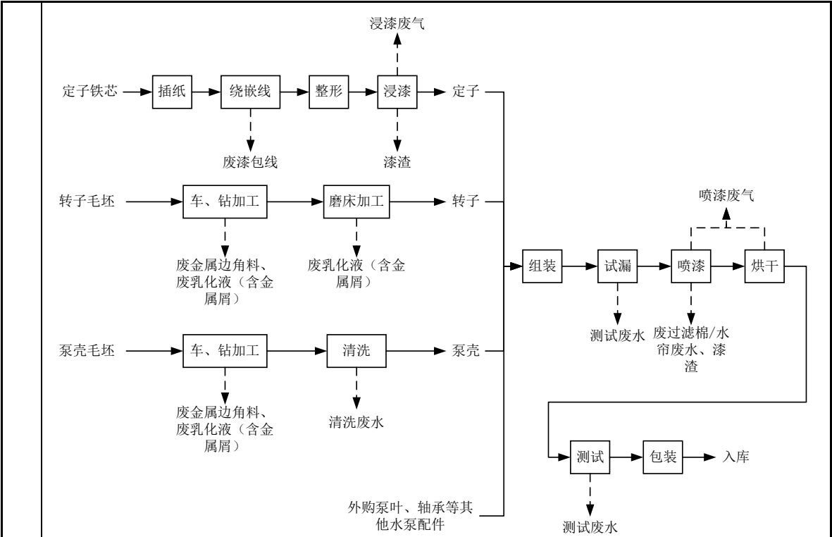
图2-2 项目水泵生产工艺及产污环节图
