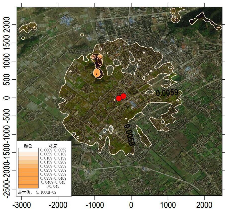
图 6.1-5 二甲苯叠加本底后小时平均浓度分布图 ( \text{mg}/\text{m}^3 )
