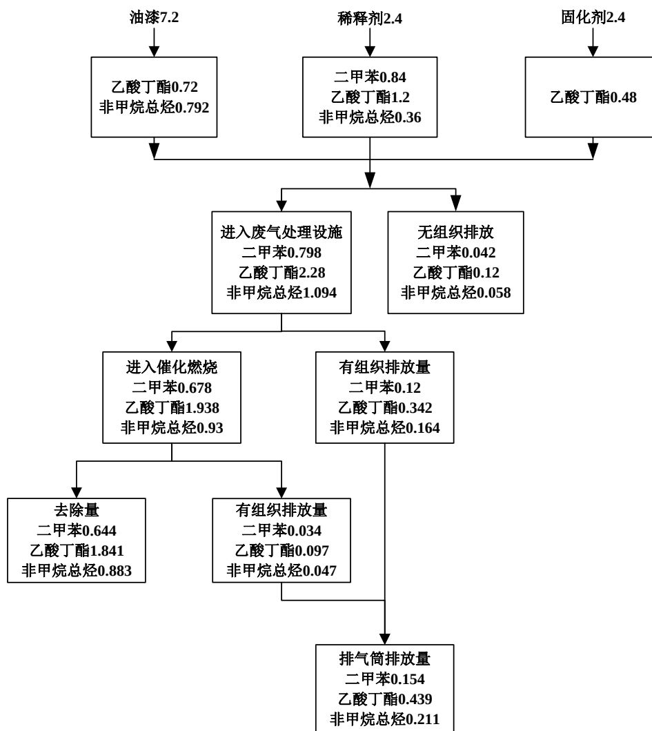
图 4.3-1 项目油性漆有机溶剂用量平衡图 单位 t/a
