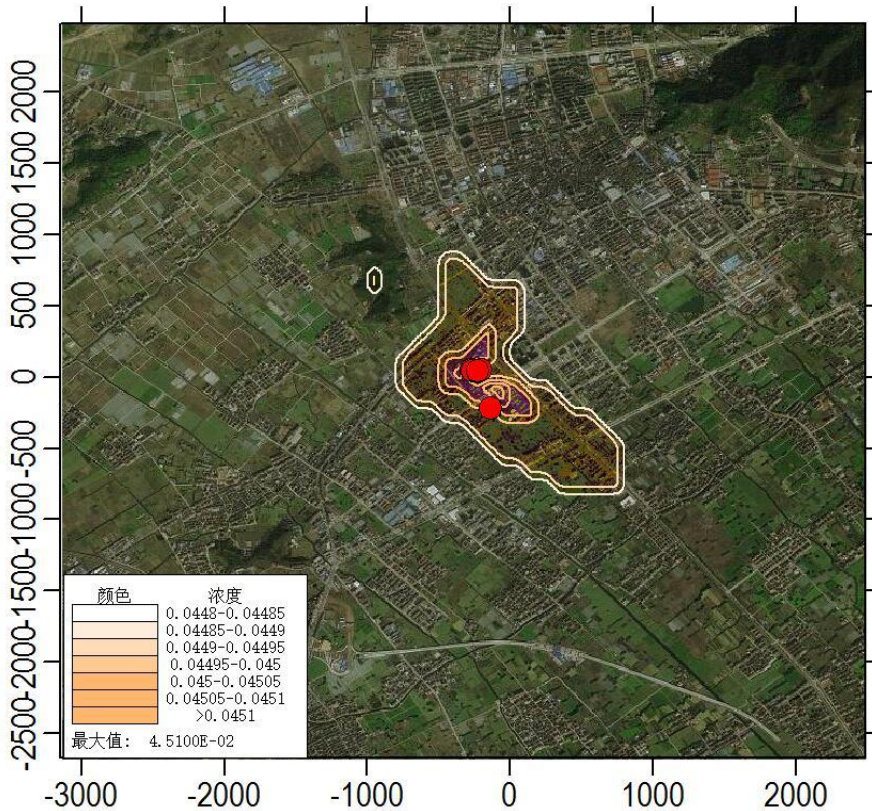
图 6.1-9 PM_{10} 叠加本底后年均浓度分布图 ( mg/m^3 )
