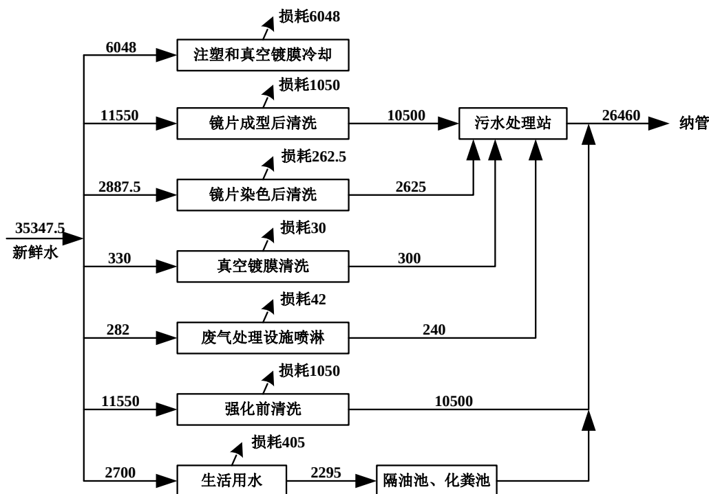
图 3.2-1 现有项目达产后水平衡图（单位：t/a）
