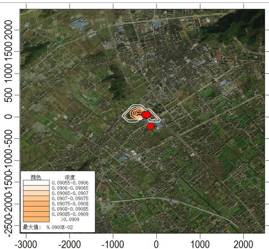
图 6.1-8 PM_{10} 叠加本底后保证率日均浓度分布图 ( mg/m^3 )
