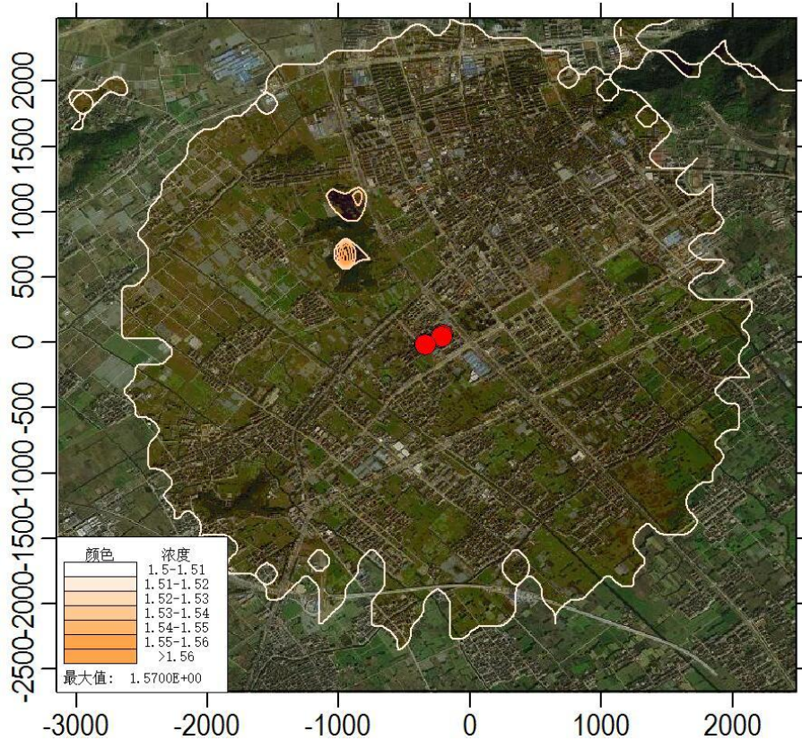
图 6.1-7 非甲烷总烃叠加本底后小时平均浓度分布图 ( \text{mg}/\text{m}^3 )
