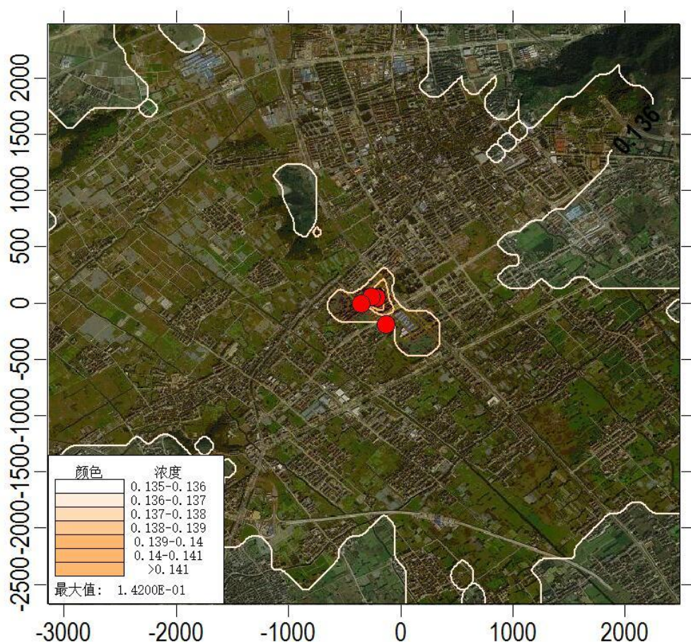
图 6.1-10 TSP 叠加本底后日均浓度分布图 (mg/m³)
