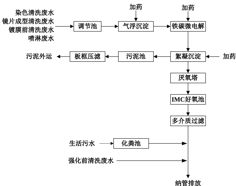
图 3.3-2 现有废水处理设施工艺流程
