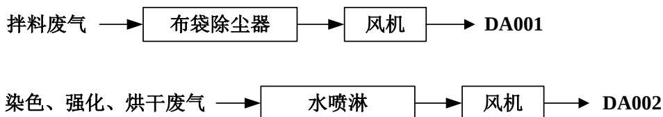
图 3.3-1 现有项目废气处理工艺流程图
