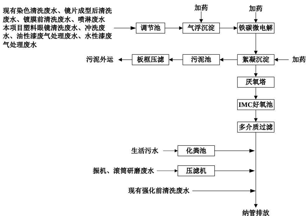
图 7.1-3 企业废水处理设施工艺流程图
