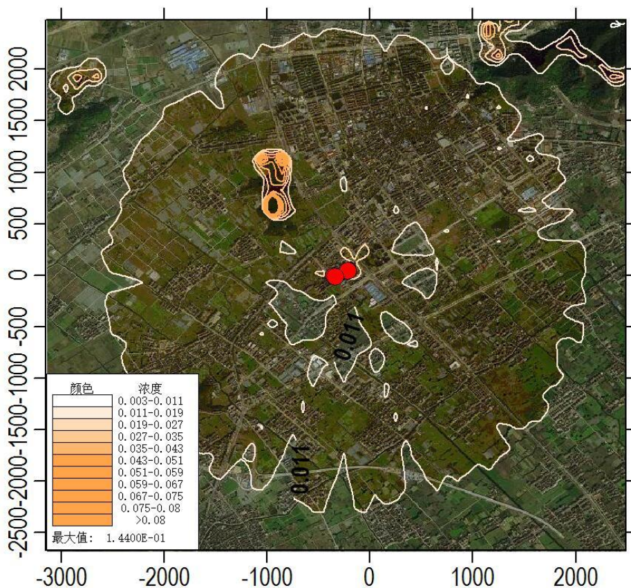
图 6.1-6 乙酸丁酯叠加本底后小时平均浓度分布图 ( \text{mg}/\text{m}^3 )
