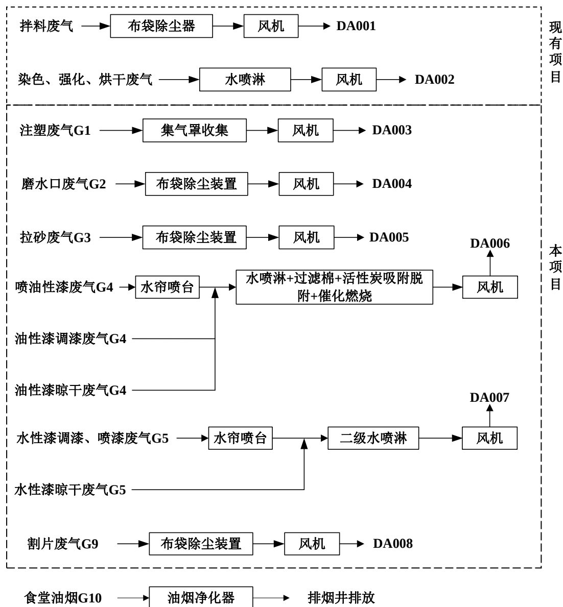
图 7.1-1 企业废气处理工艺流程图
