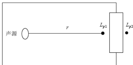
图 6.1-11 室内声源等效为室外声源图例
