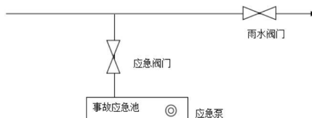
图 6.1-12 事故废水（消防废水）收集系统示意图
