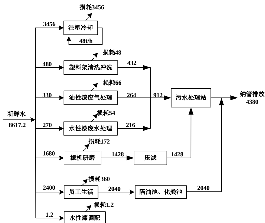
图 4.3-3 项目水平衡图 单位:t/a
