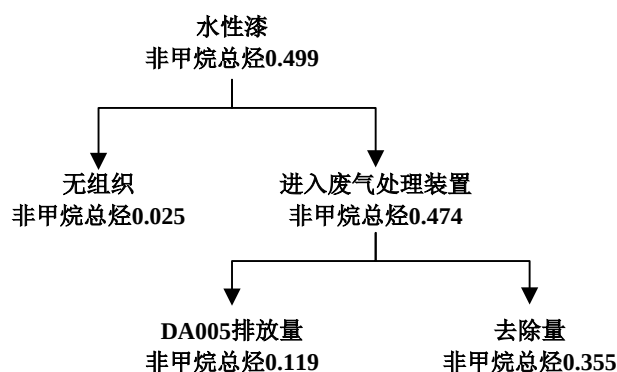
图 4.3-2 项目水性漆有机溶剂用量平衡图 单位 t/a
