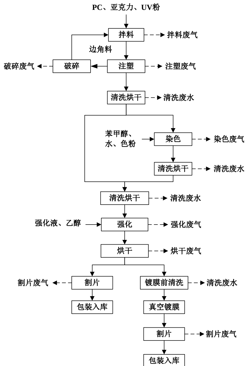
图 3.1-1 现有眼镜片生产工艺流程图
