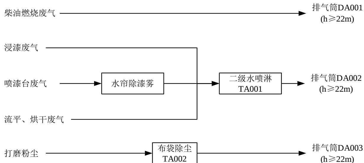
图4-1 废气处理工艺流程图
