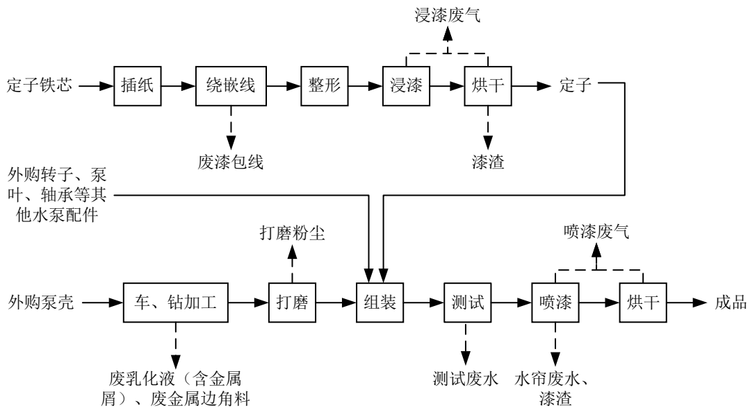
图2-2 项目水泵生产工艺及产污环节图
