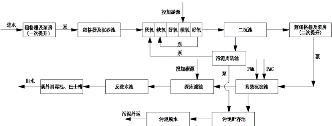
图 4-2 二期污水处理工艺流程图
