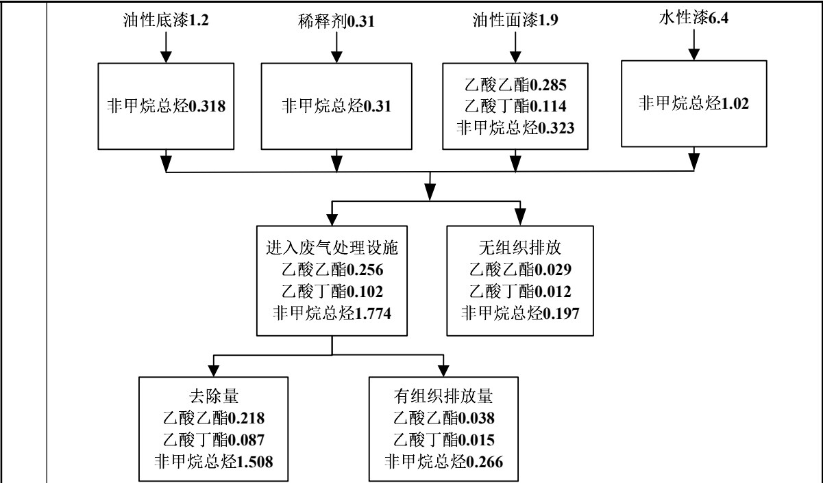
图 2-2 涂料有机溶剂平衡图 单位 t/a
