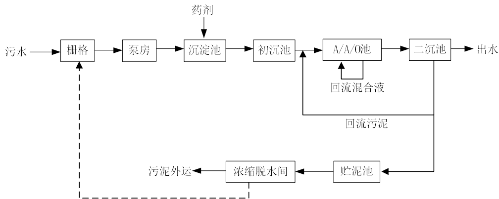
图 4-3 A/A/O 工艺流程
