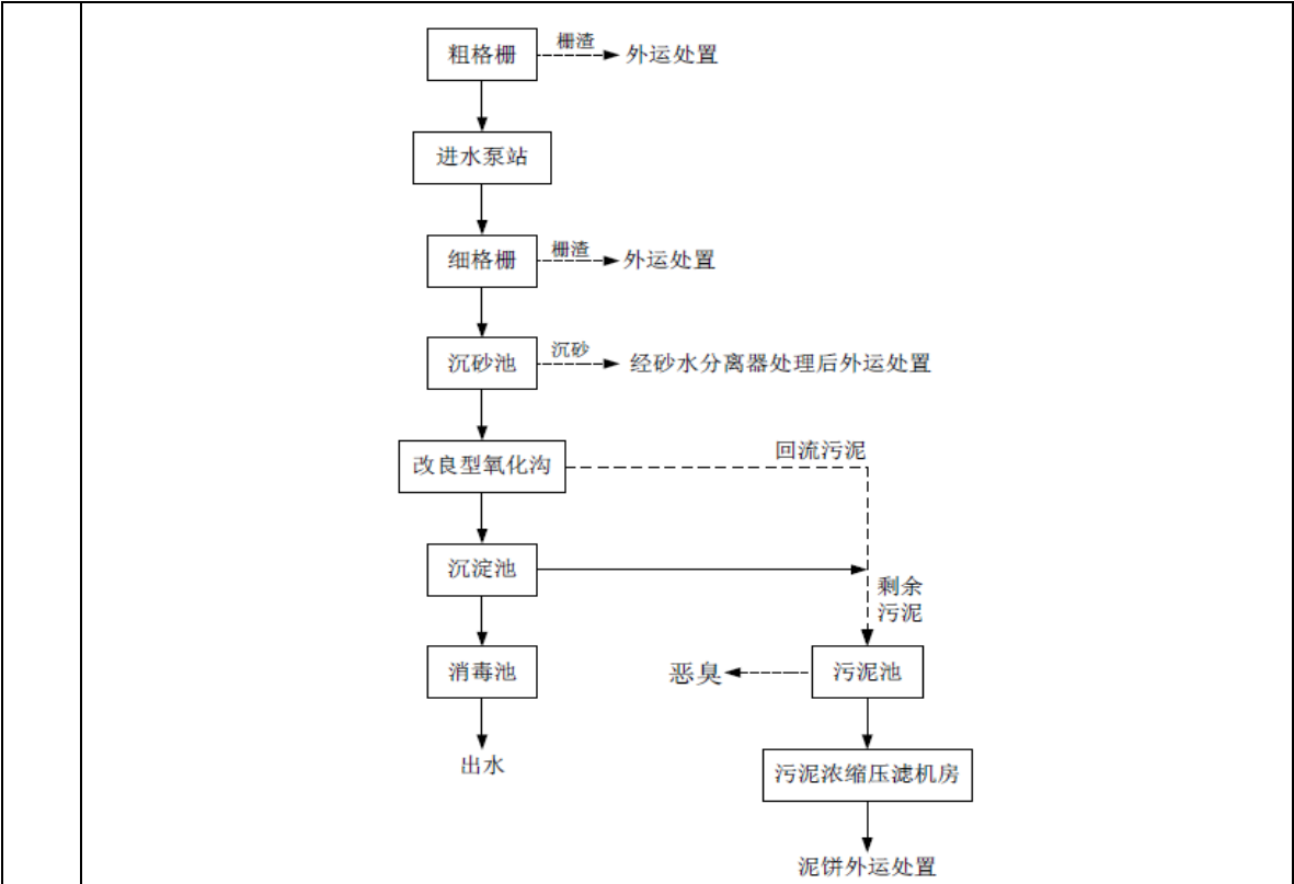
图4-4 一期污水处理工艺流程图
