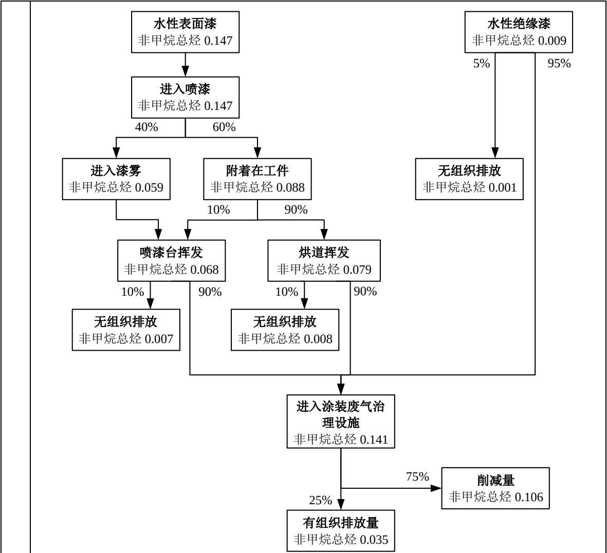
图2-2 水性表面漆、水性绝缘漆溶剂平衡图 单位：t/a
