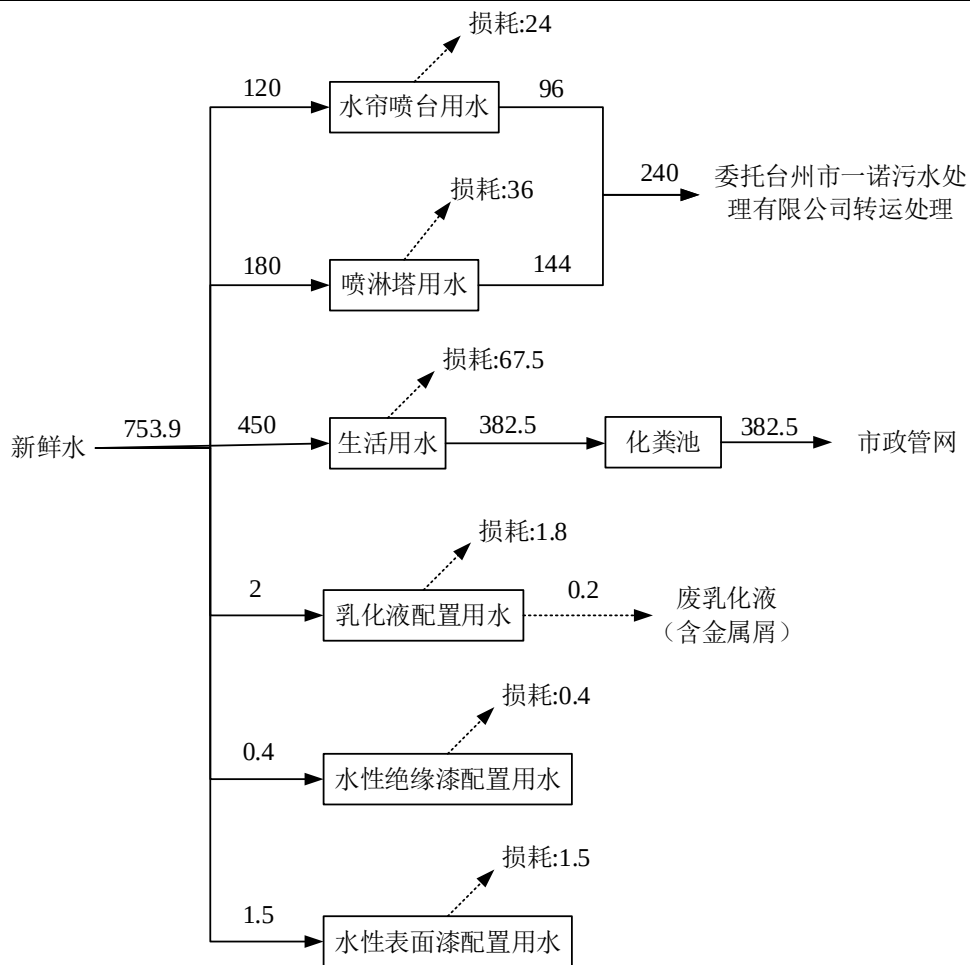
图2-1 水平衡图 (t/a)
