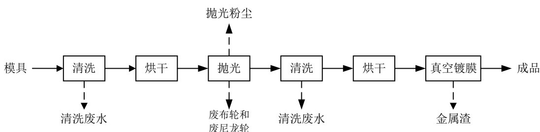
图2-3 项目模具生产工艺及产污环节图
