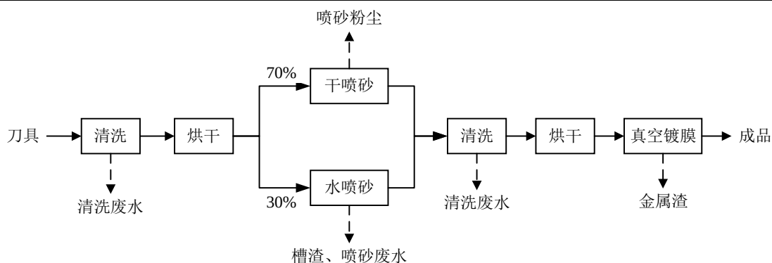
图2-2 项目杆装刀具生产工艺及产污环节图
