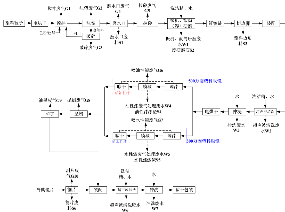
图 3.2-1 项目生产工艺流程图
