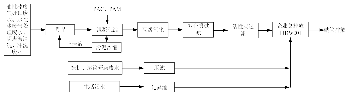
图 6.1-3 项目污水处理工艺图
