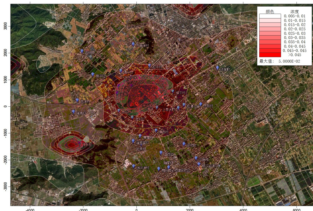
图 5.1-7 乙酸乙酯叠加本底后+同类源小时平均浓度分布图 ( \text{mg}/\text{m}^3 )
