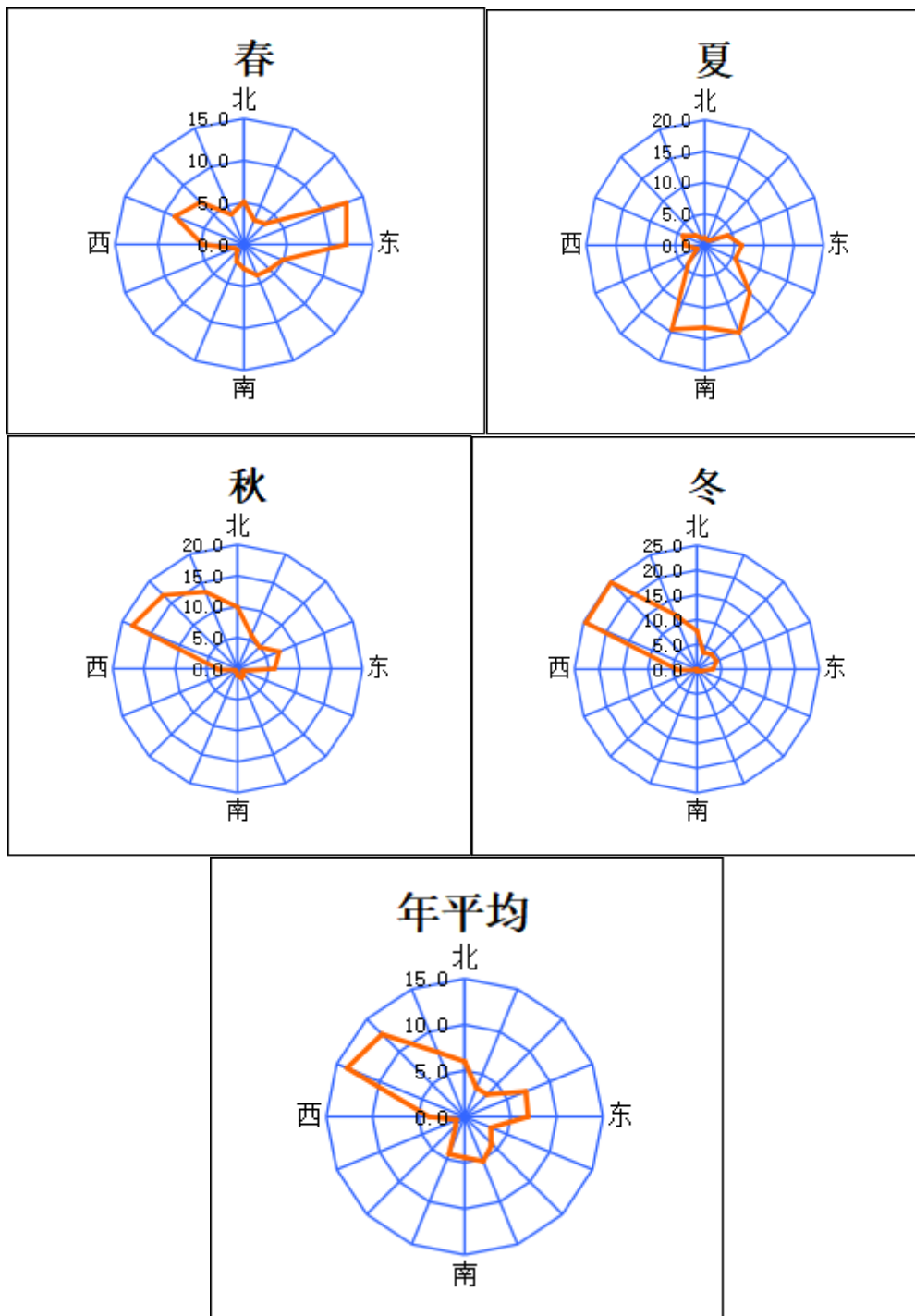
图 5.1-4 风向玫瑰图
