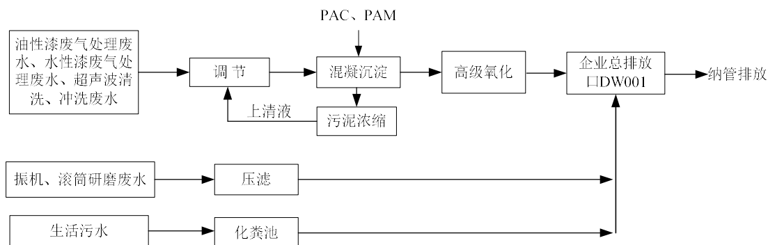
图 6.1-3 项目污水处理工艺图
