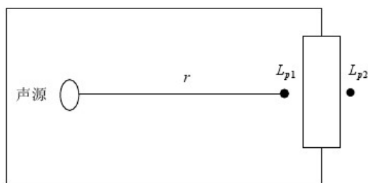
图 5.1-11 室内声源等效为室外声源图例
