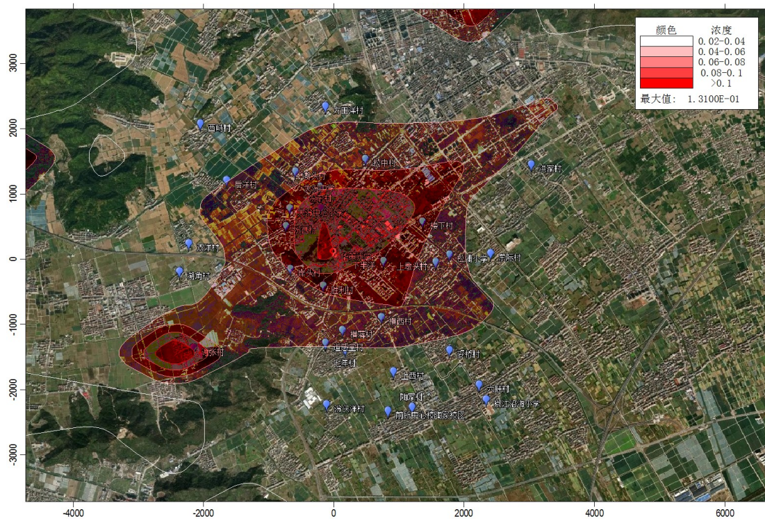
图 5.1-8 乙酸丁酯叠加本底后+同类源小时平均浓度分布图 ( \text{mg}/\text{m}^3 )
