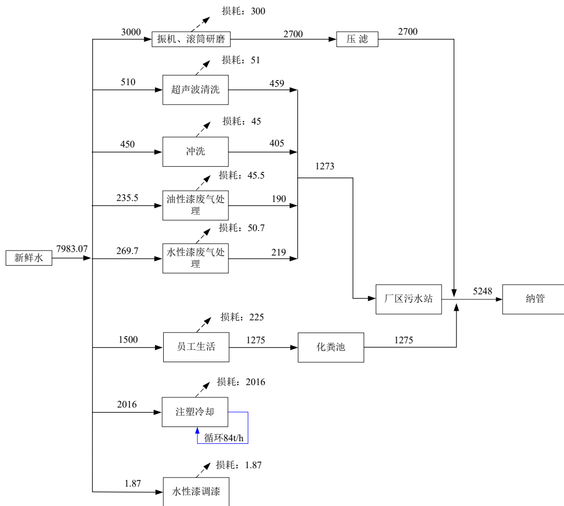
图 3.3-2 项目水平衡图 单位:t/a
