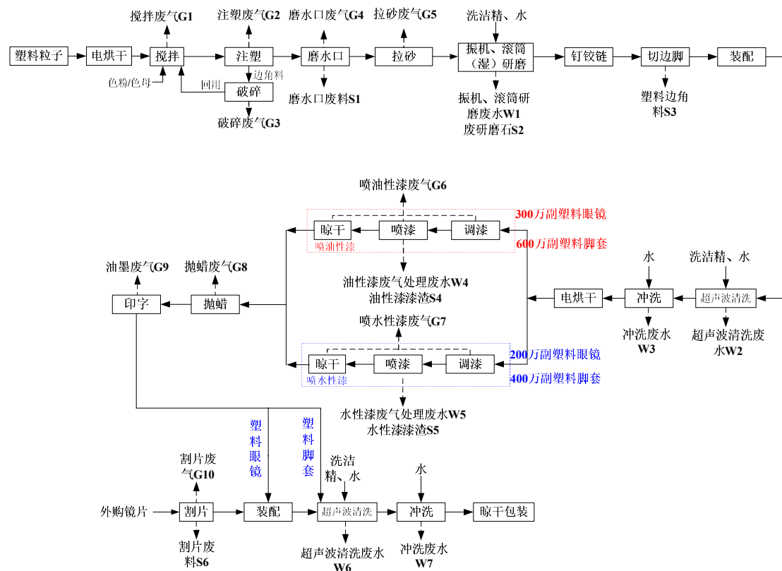
图 3.2-1 项目生产工艺流程图
