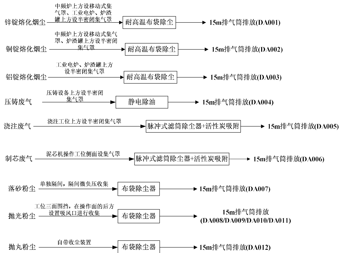
图 7-3 废气处理工艺流程图
