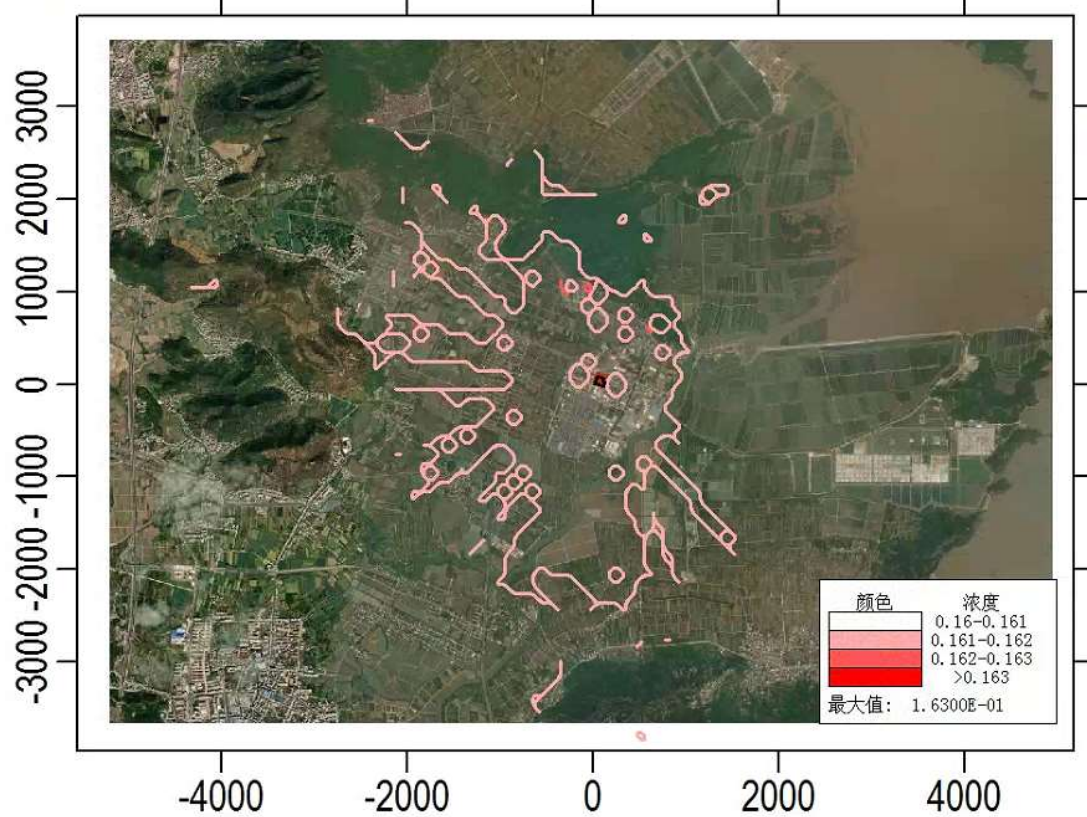
叠加背景浓度、其他在建、拟建污染源后氨小时浓度最大值分布图 ( \text{mg}/\text{m}^3 )
