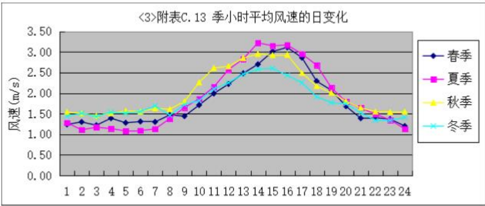
图 7-6 季小时平均风速的日变化曲线
