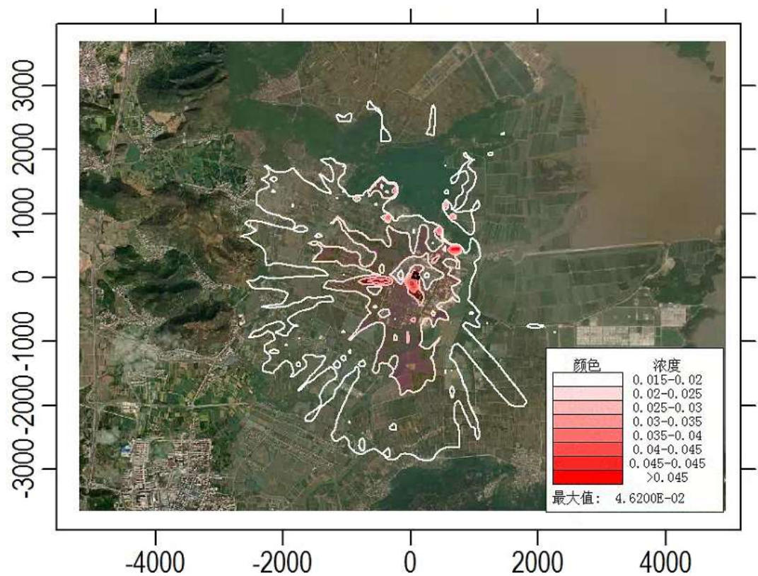
非正常工况下苯酚小时浓度最大值分布图 ( \text{mg}/\text{m}^3 )
