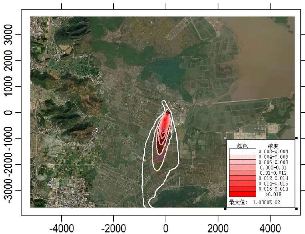
TSP 年均贡献浓度最大值分布图 ( \text{mg}/\text{m}^3 )
