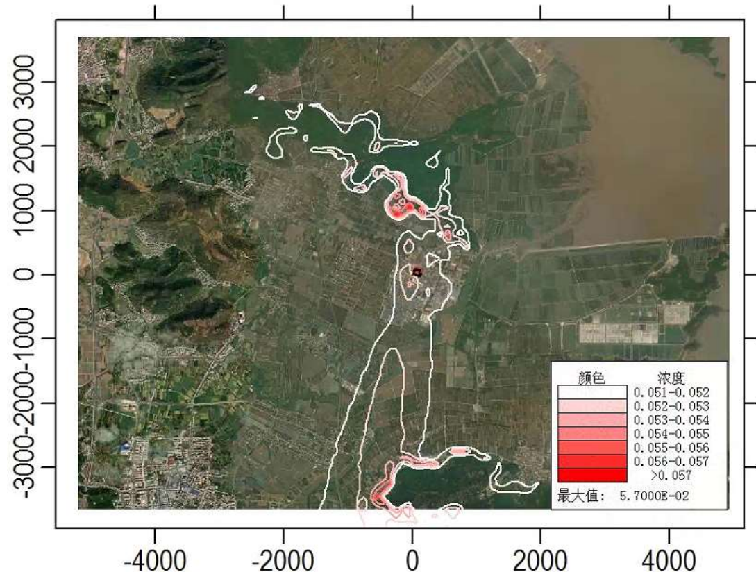
叠加背景浓度、其他在建、拟建污染源后 PM 2.5 保证率日均浓度最大值分布图 (mg/m³)
