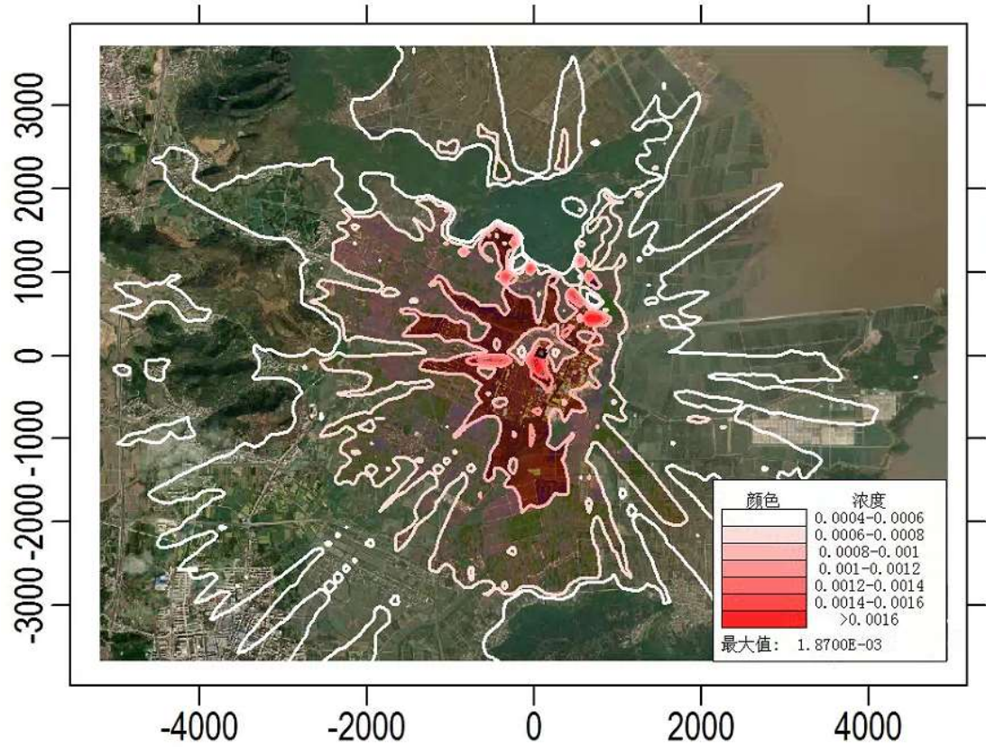
甲醛小时贡献浓度最大值分布图 (mg/m 3 )
