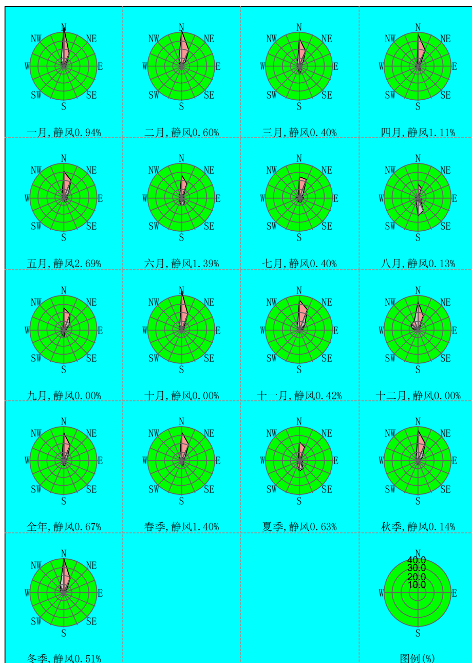
图 7-7 风向玫瑰图
