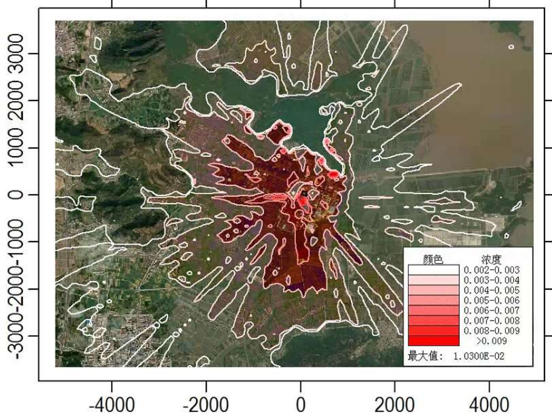
非正常工况下甲醛小时浓度最大值分布图 ( \text{mg}/\text{m}^3 )
