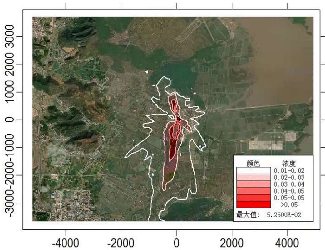
TSP 日均贡献浓度最大值分布图 ( \text{mg}/\text{m}^3 )
