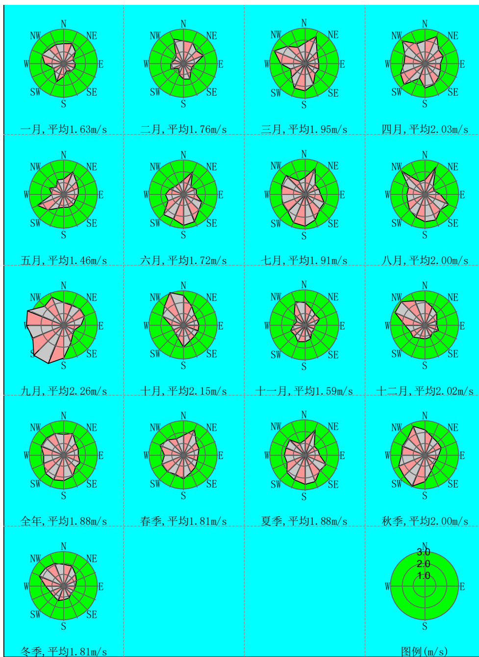
图 7-8 风速玫瑰图
