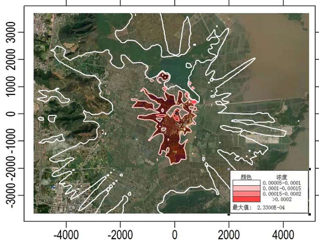
铅及其化合物小时贡献浓度最大值分布图 ( \text{mg}/\text{m}^3 )
