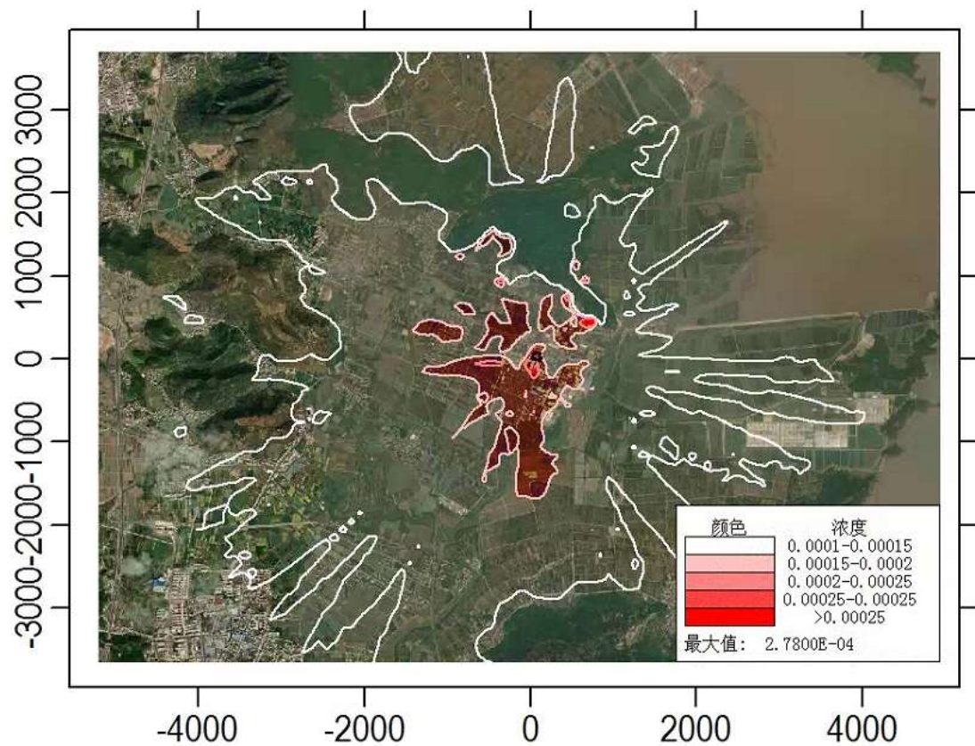
叠加背景浓度、其他在建、拟建污染源后铅及其化合物小时浓度最大值分布图 ( \text{mg}/\text{m}^3 )
