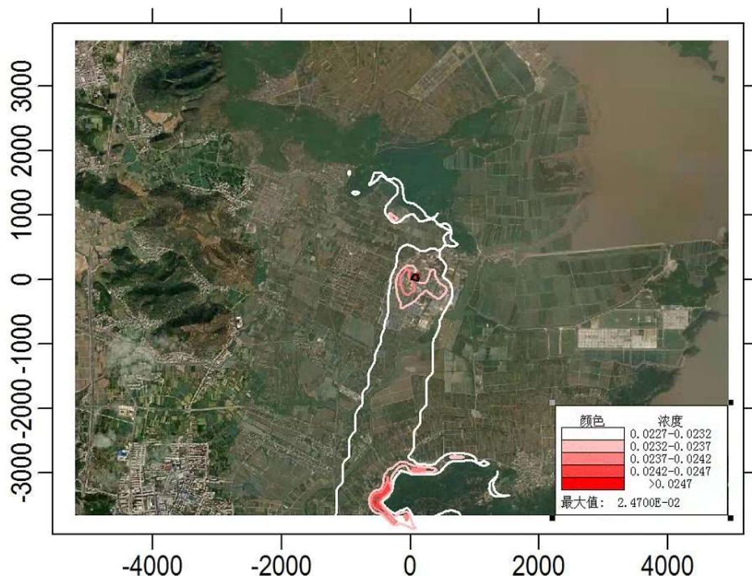
叠加背景浓度、其他在建、拟建污染源后 PM_{2.5} 年均浓度最大值分布图 ( mg/m^3 )
