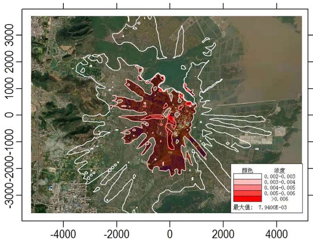
非正常工况下氨小时浓度最大值分布图 ( \text{mg}/\text{m}^3 )
