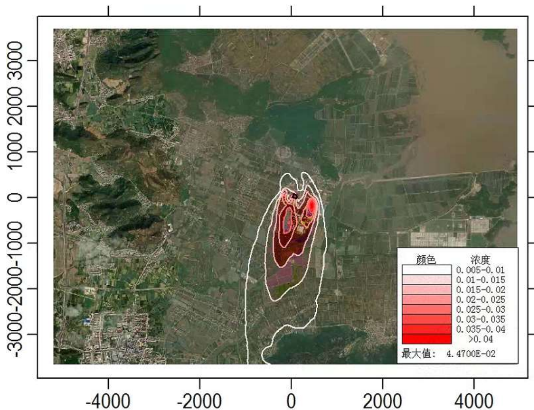
叠加其他在建、拟建污染源后 TSP 年均浓度最大值分布图 (mg/m³)
