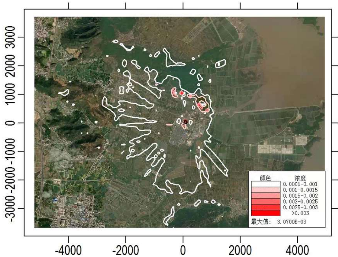
氨小时贡献浓度最大值分布图 ( \text{mg}/\text{m}^3 )
