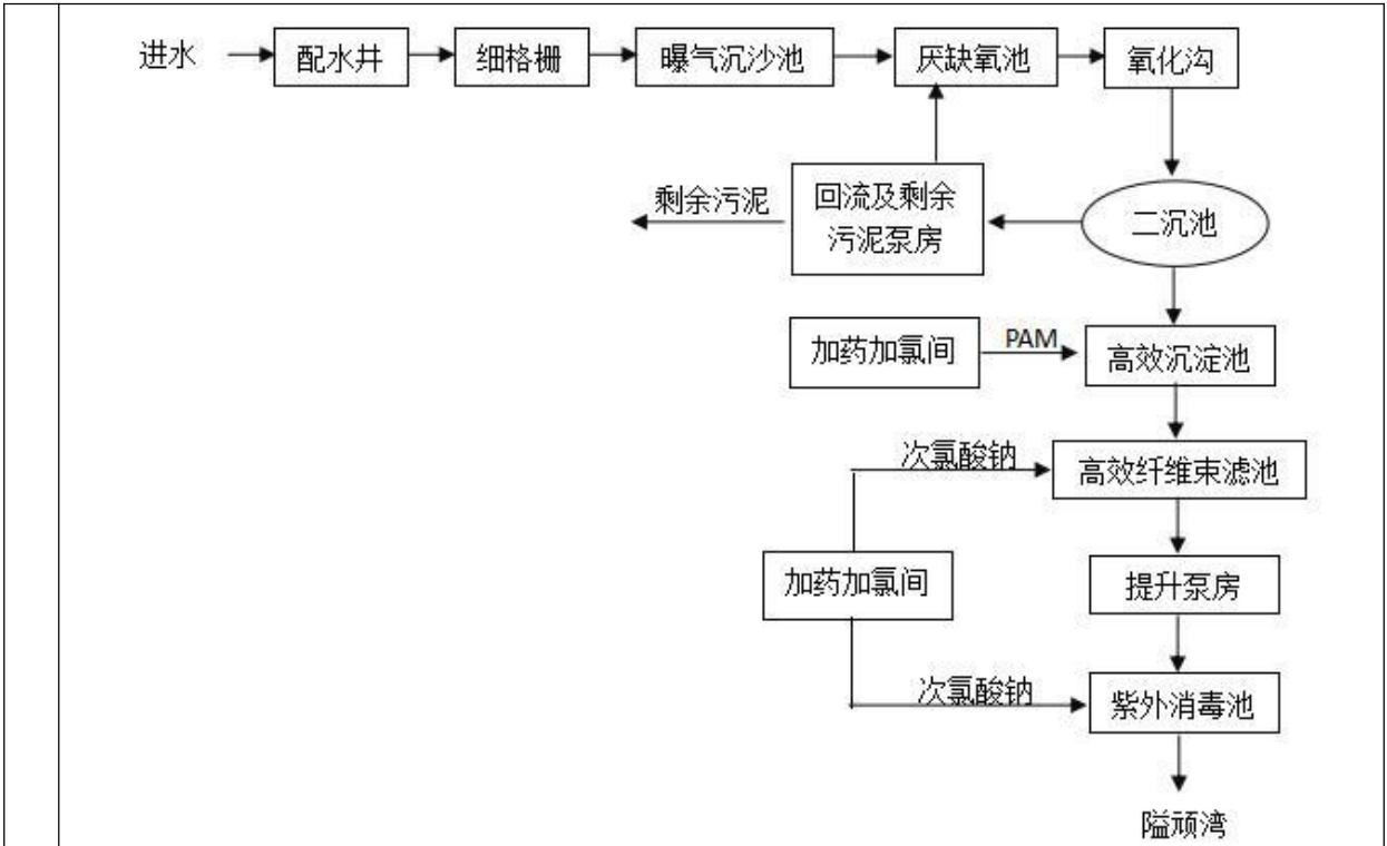
图 4-4 温岭市观岙污水处理厂一期提标工程工艺流程图
