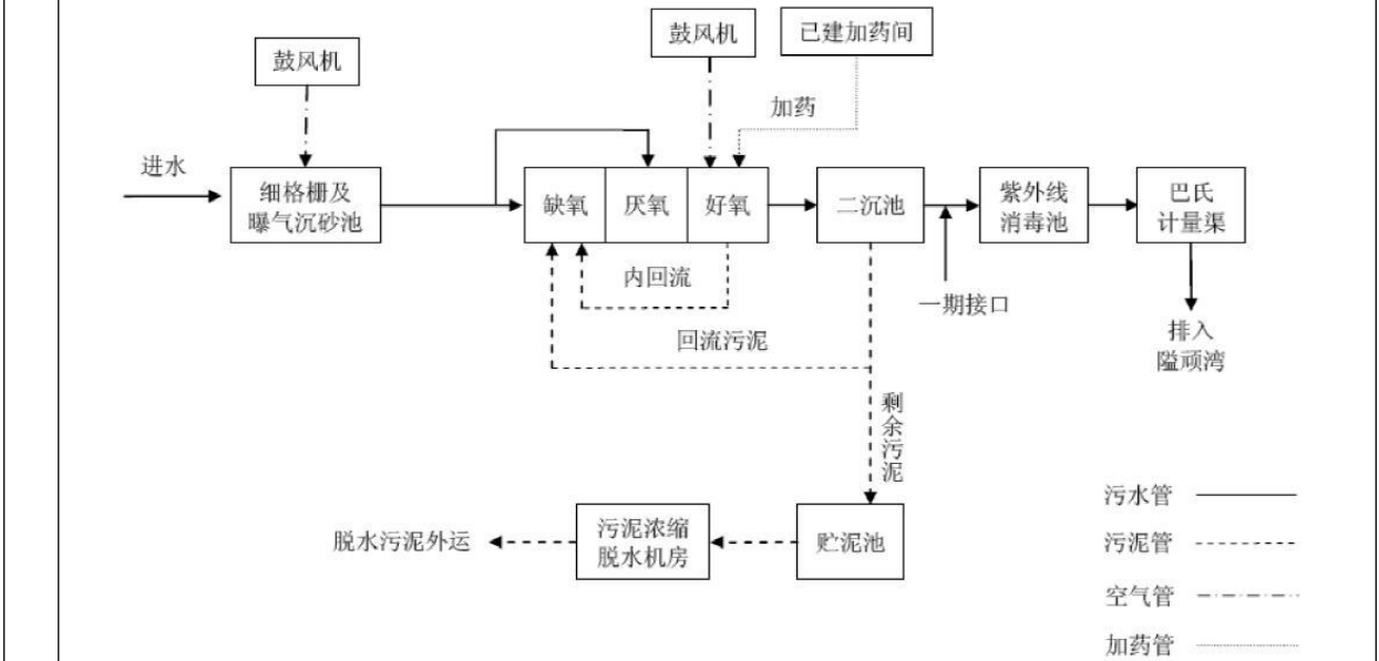
图 4-5 温岭市观岙污水处理厂二期工程工艺流程图
