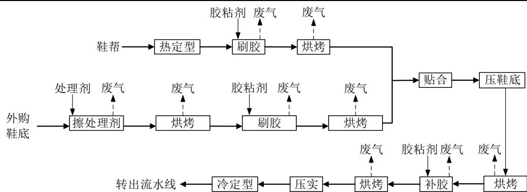
图 2-4 冷粘流水线生产工艺流程及产污环节细化图
