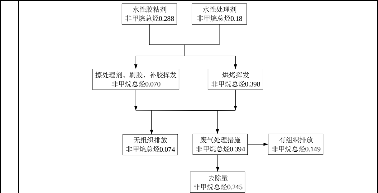
图 2-1 水性胶粘剂、处理剂有机挥发物平衡图 单位：t/a
