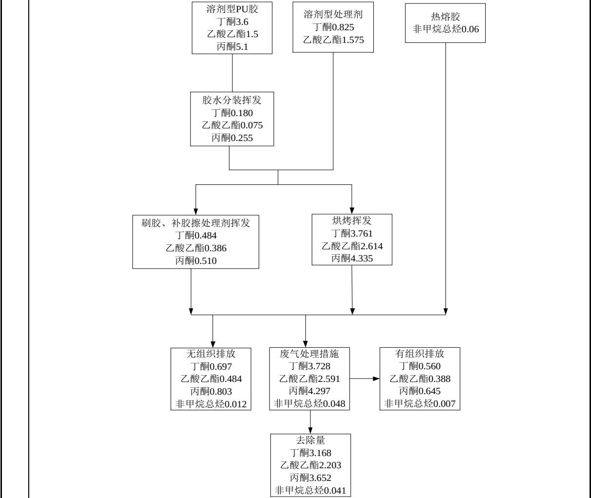
图 2-2 热熔胶、溶剂型 PU 胶、处理剂有机挥发物平衡图 单位：t/a
