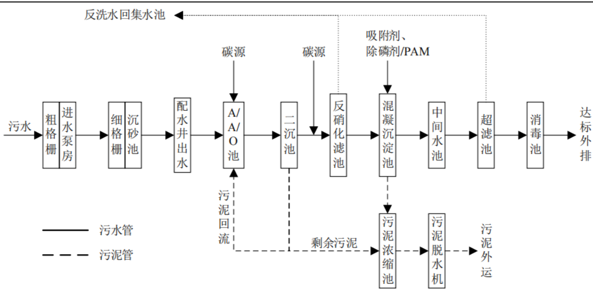
图 4-3 温岭市新河镇污水处理厂废水处理工艺流程图
