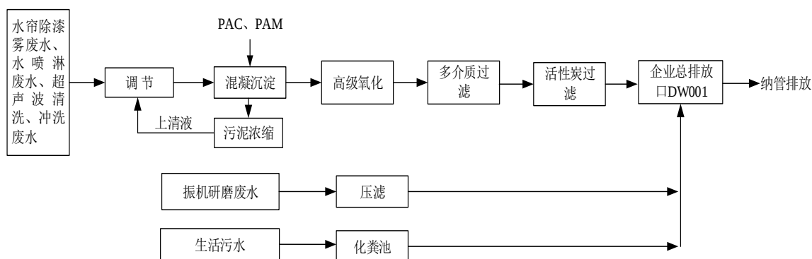
图 6.1-3 企业废水处理设施工艺流程图
