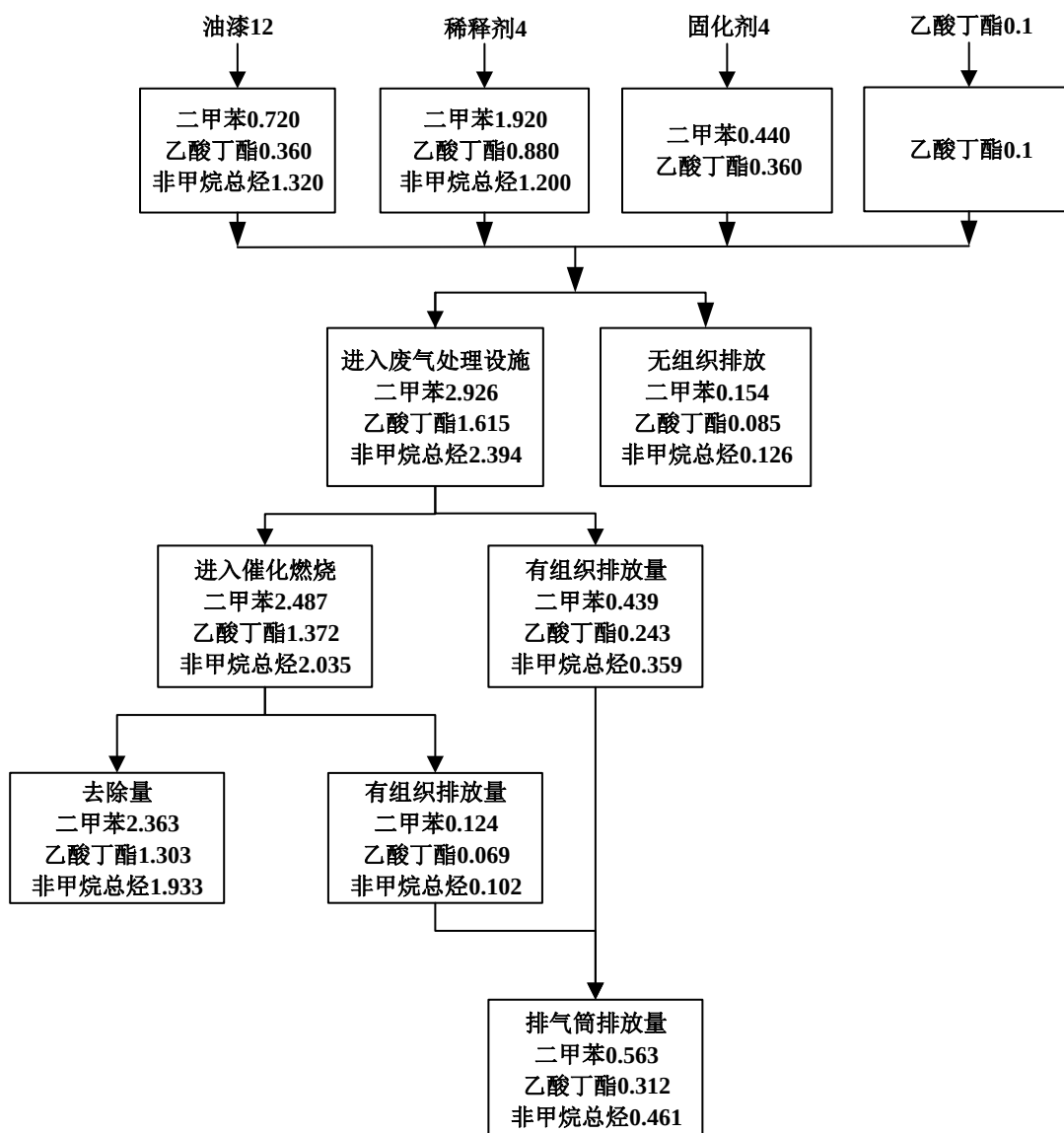
图 3.3-1 项目油性漆涂装过程有机溶剂用量平衡图 单位 t/a
