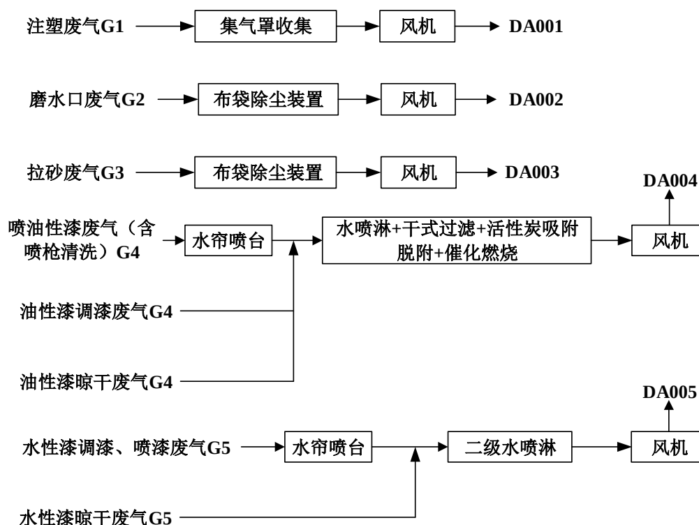
图 6.1-1 企业废气处理工艺流程图
