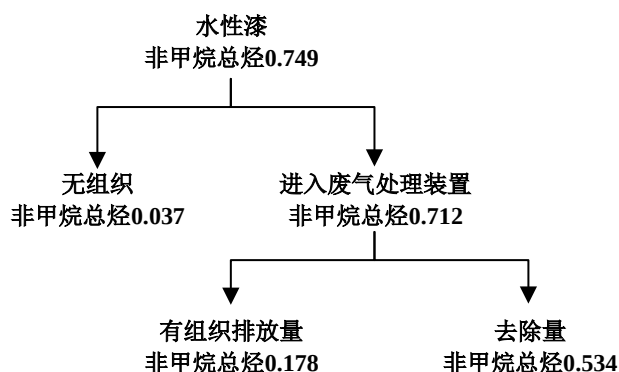
图 3.3-2 项目水性漆有机溶剂用量平衡图 单位 t/a
