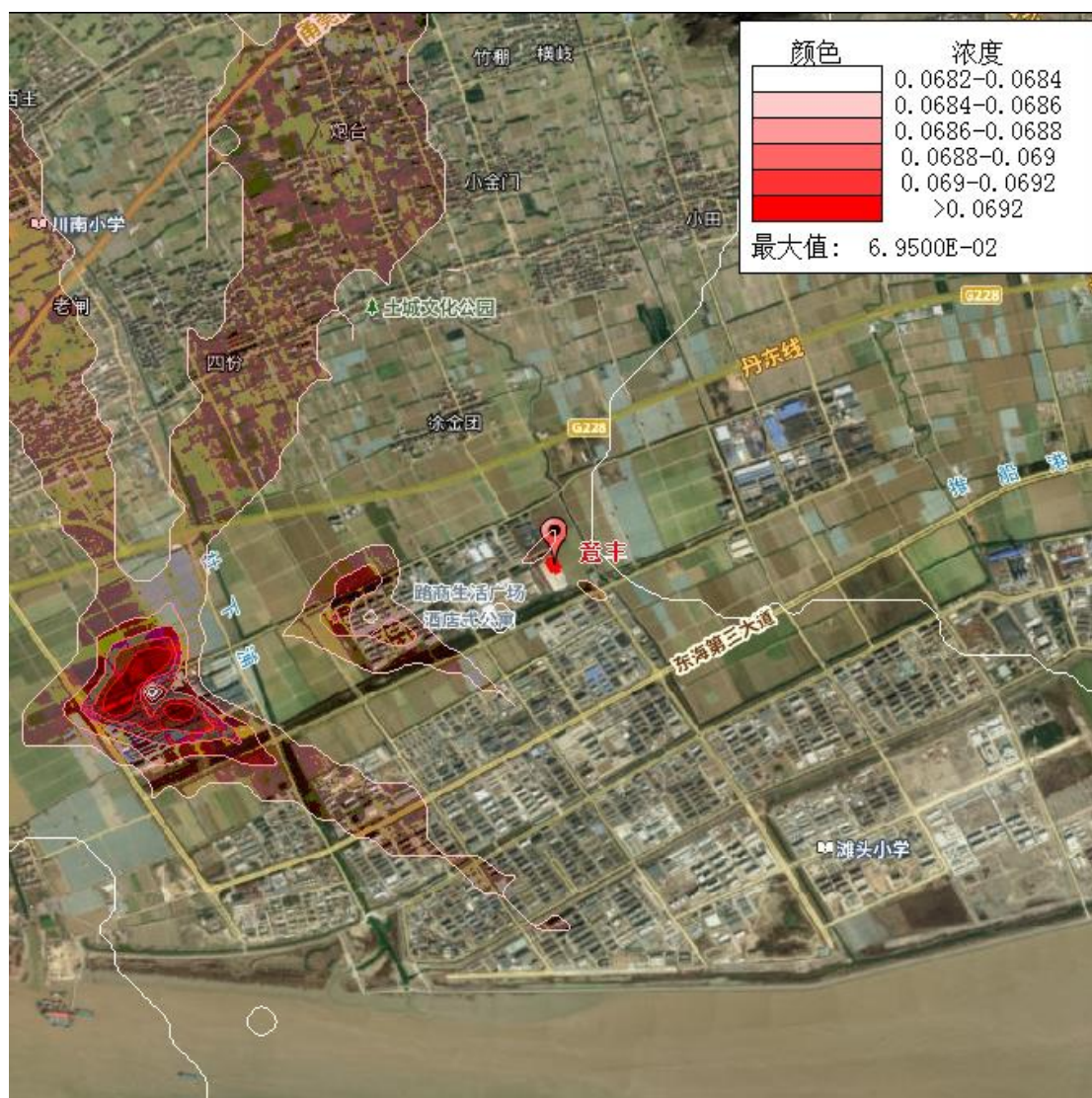
图 5.1-8 PM_{10} 叠加本底后保证率日均浓度分布图 ( mg/m^3 )
