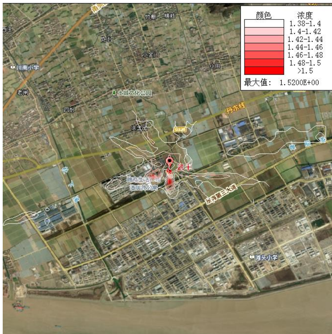
图 5.1-7 非甲烷总烃叠加本底后小时平均浓度分布图 ( \text{mg}/\text{m}^3 )
