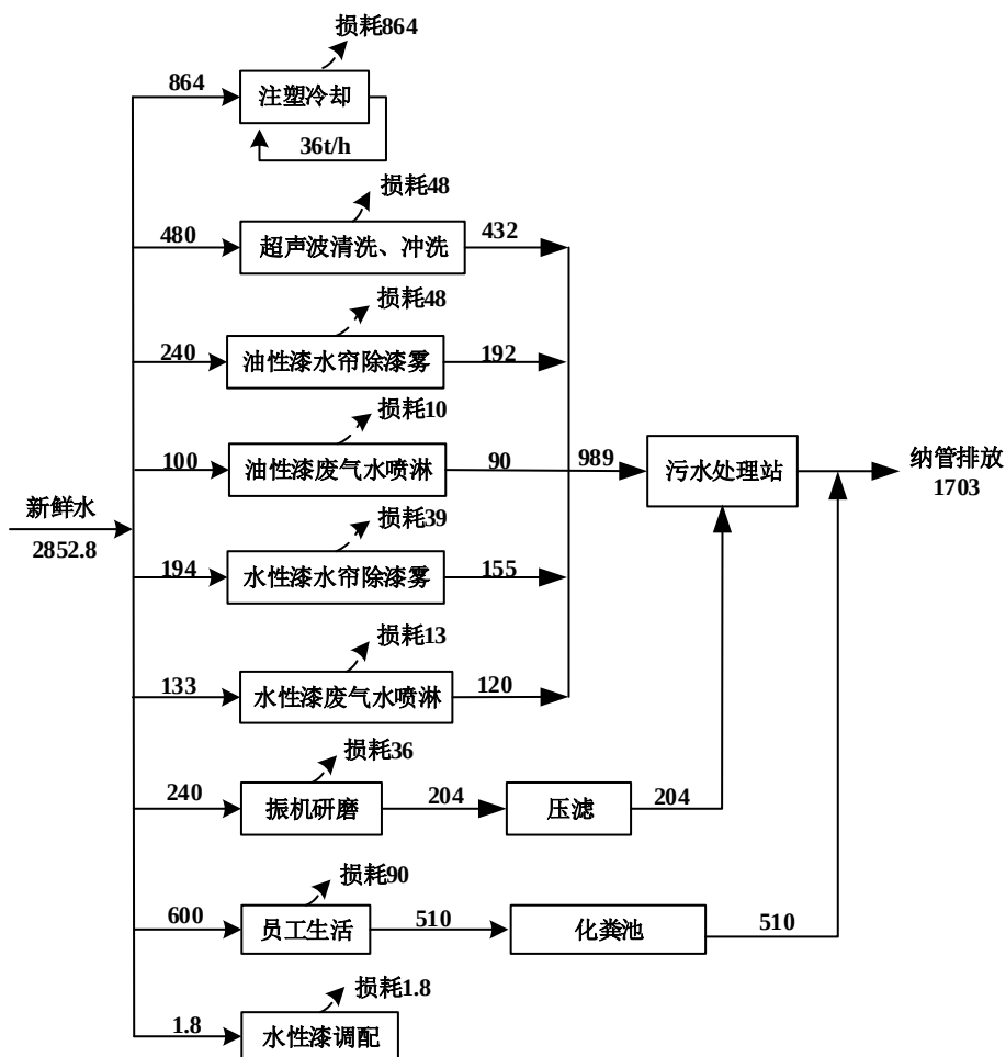
图 3.3-3 项目水平衡图 单位:t/a
