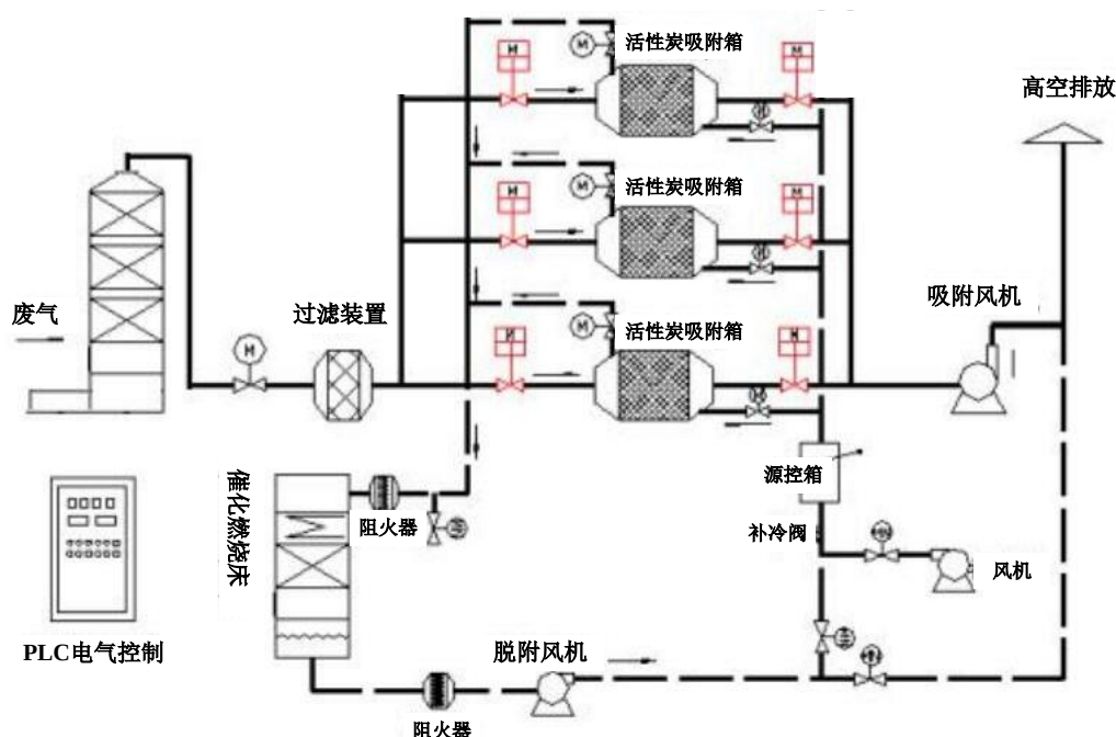
图 6.1-2 油性漆涂装废气处理工艺
