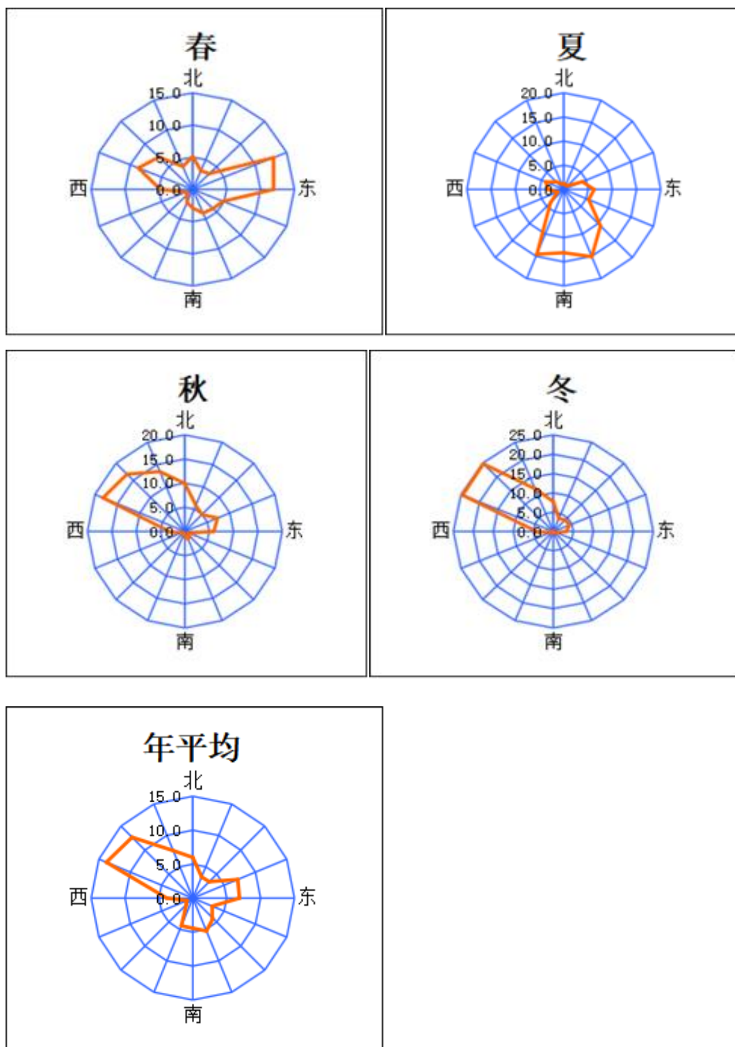
图 5.1-4 风向玫瑰图
