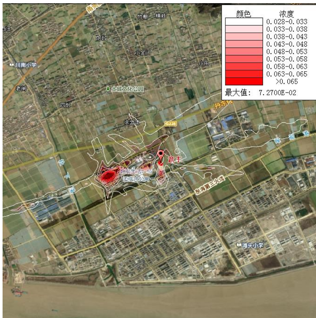
图 5.1-6 乙酸丁酯叠加本底后小时平均浓度分布图 ( \text{mg}/\text{m}^3 )
