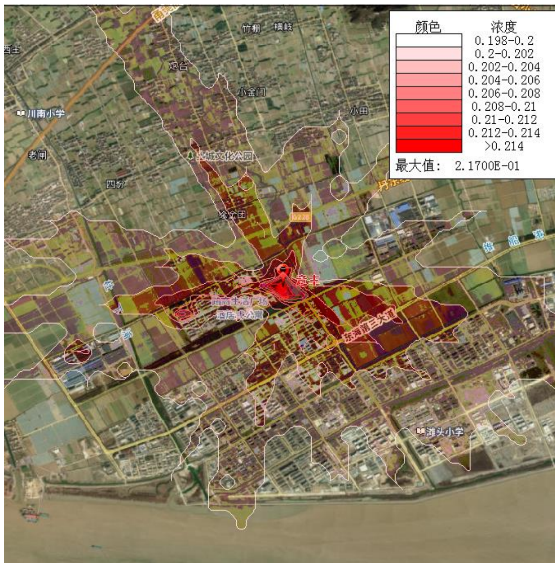
图 5.1-10 TSP 叠加本底后日均浓度分布图 (mg/m³)
