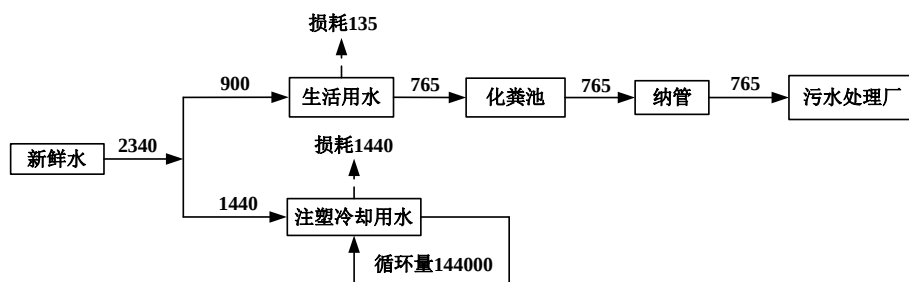
图 2-1 水平衡图 单位: t/a
