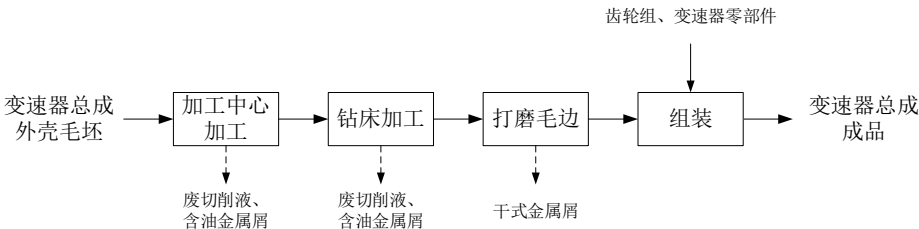
图 2-3 变速器总成生产工艺流程图
