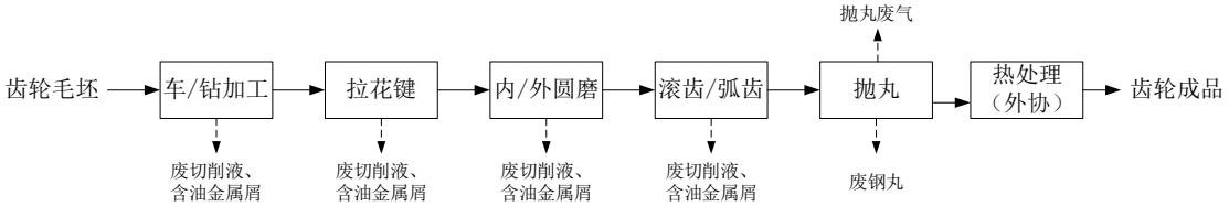
图 2-2 齿轮生产工艺流程图
