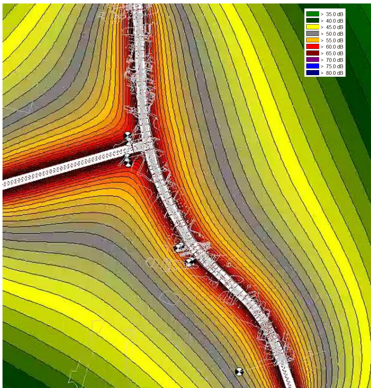
图 8-1 近期昼间交通噪声水平等声级线图
