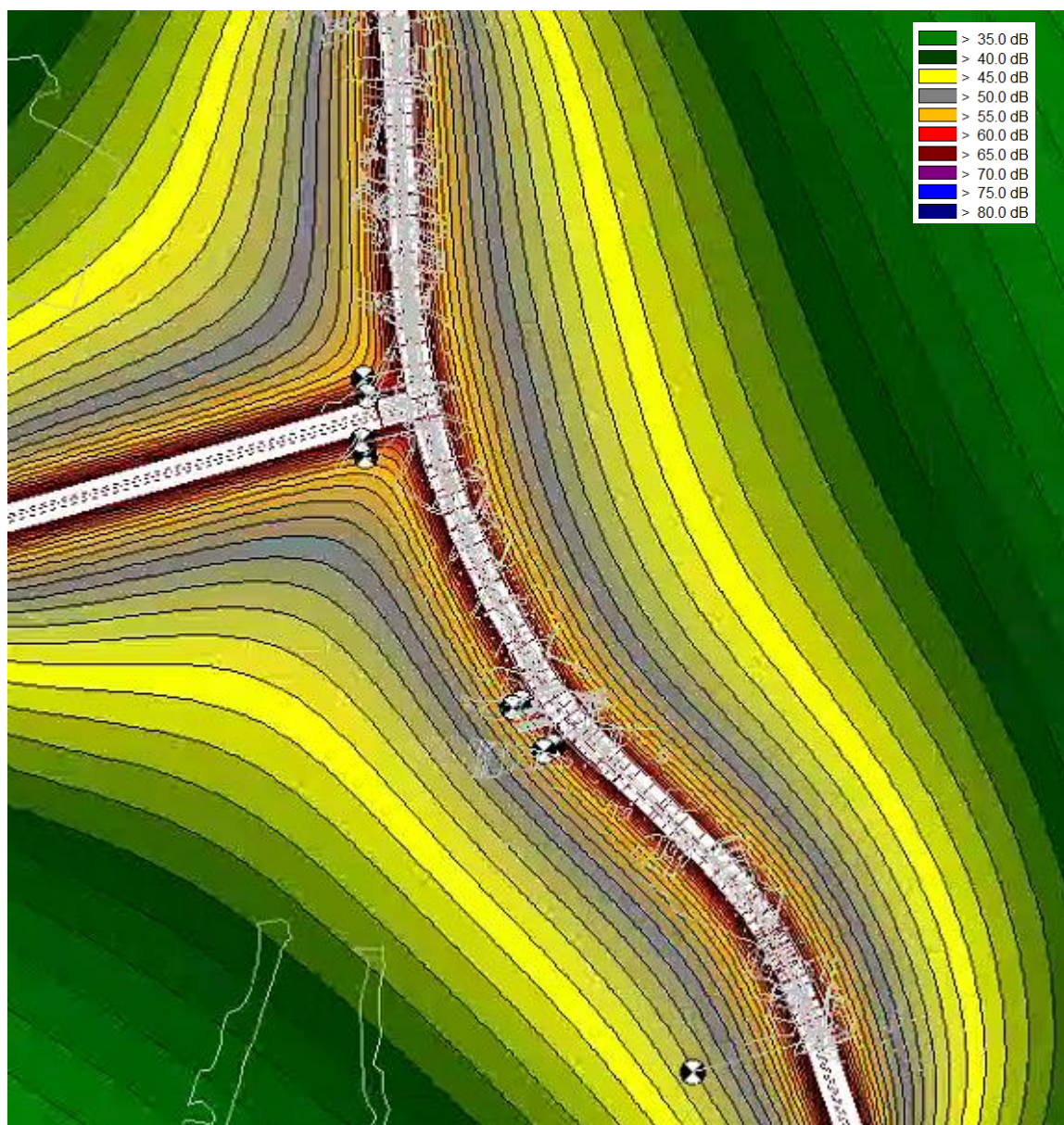
图 8-4 中期夜间交通噪声水平等声级线图
