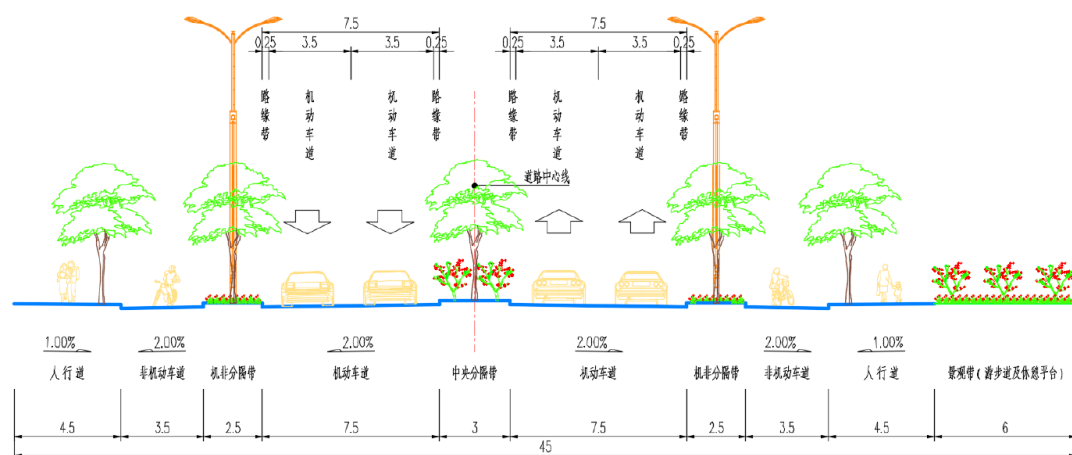
图 2-1 道路标准横断面
