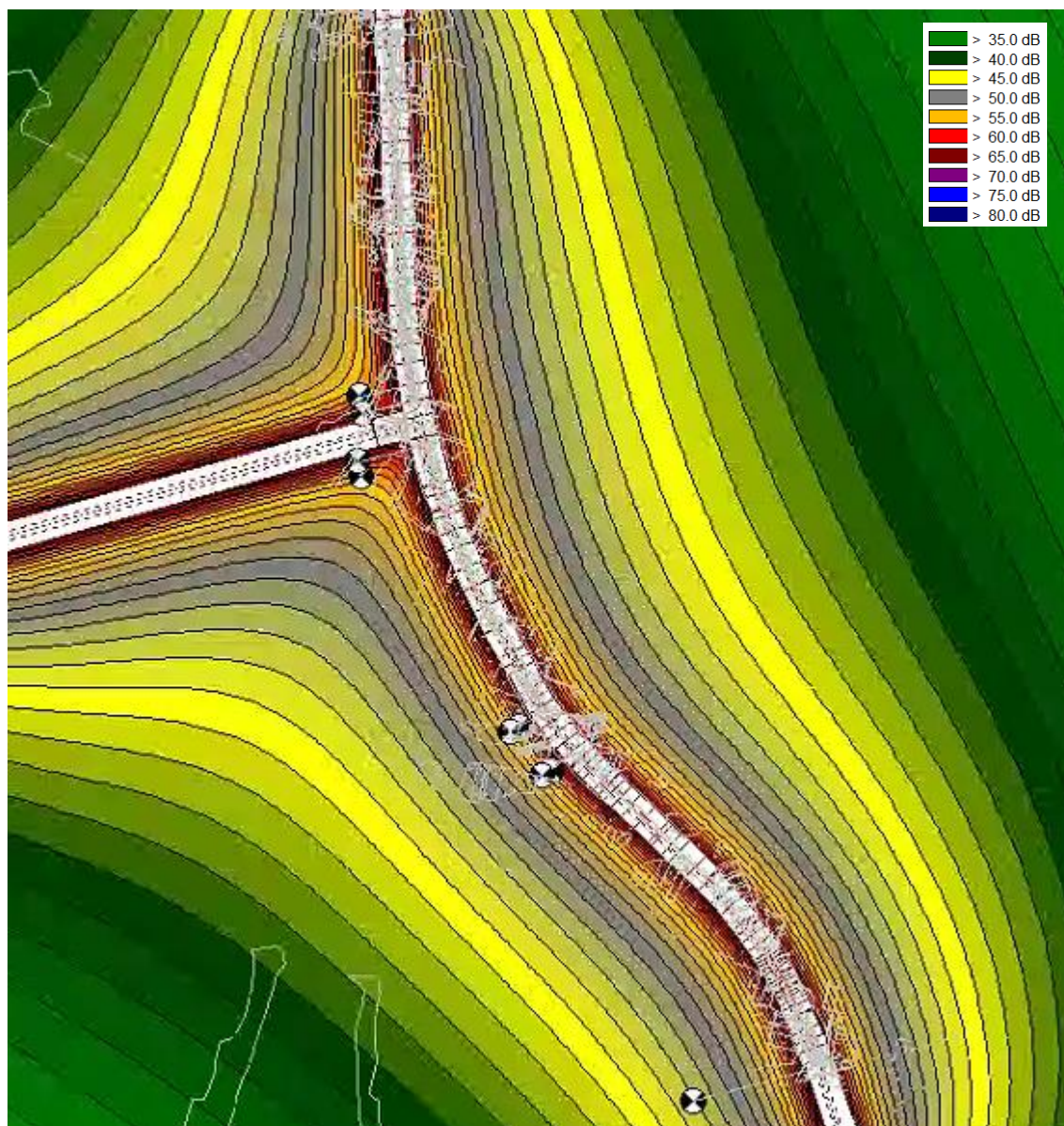
图 8-2 近期夜间交通噪声水平等声级线图
