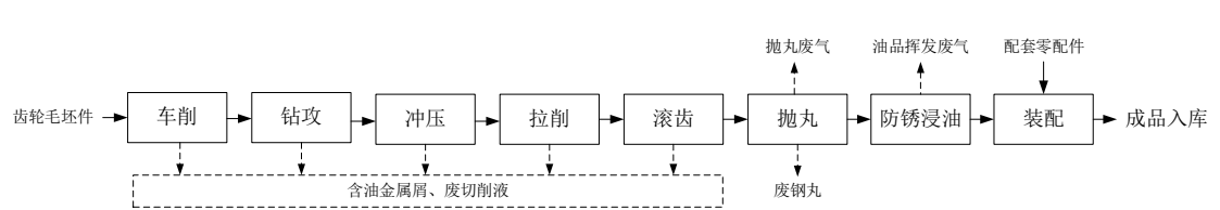
图 2-2 齿轮生产工艺流程图
