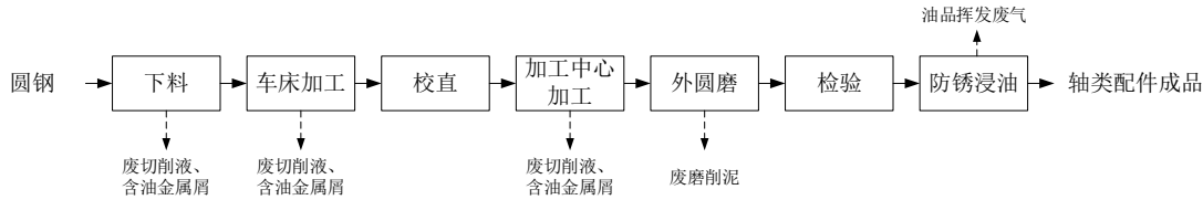
图 2-3 轴类配件生产工艺流程图
