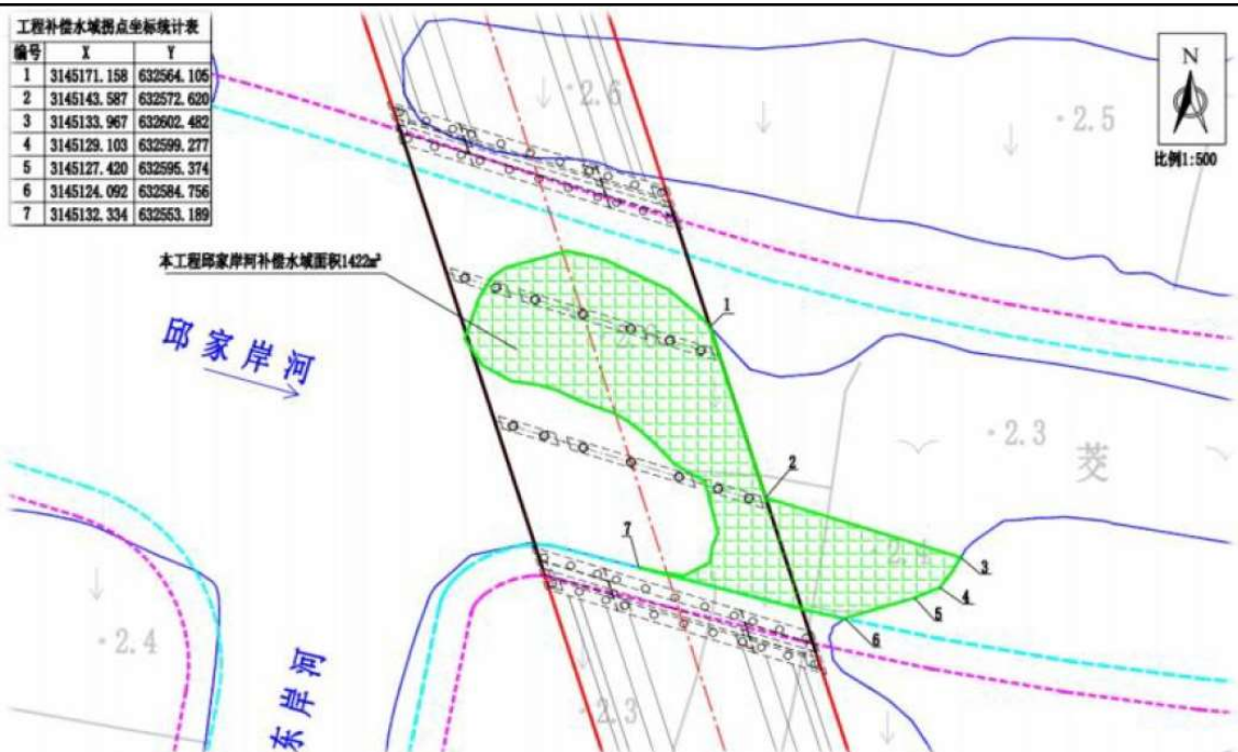
图 2-4 项目工程邱家岸河处补偿水域平面图
