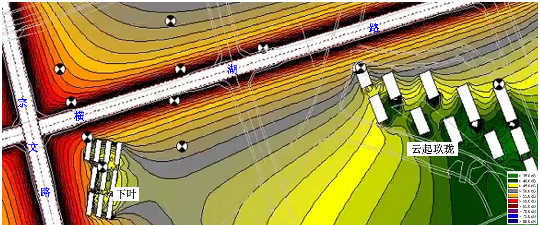
营运远期（2041年）昼间噪声等声级线图（本项目贡献值）
