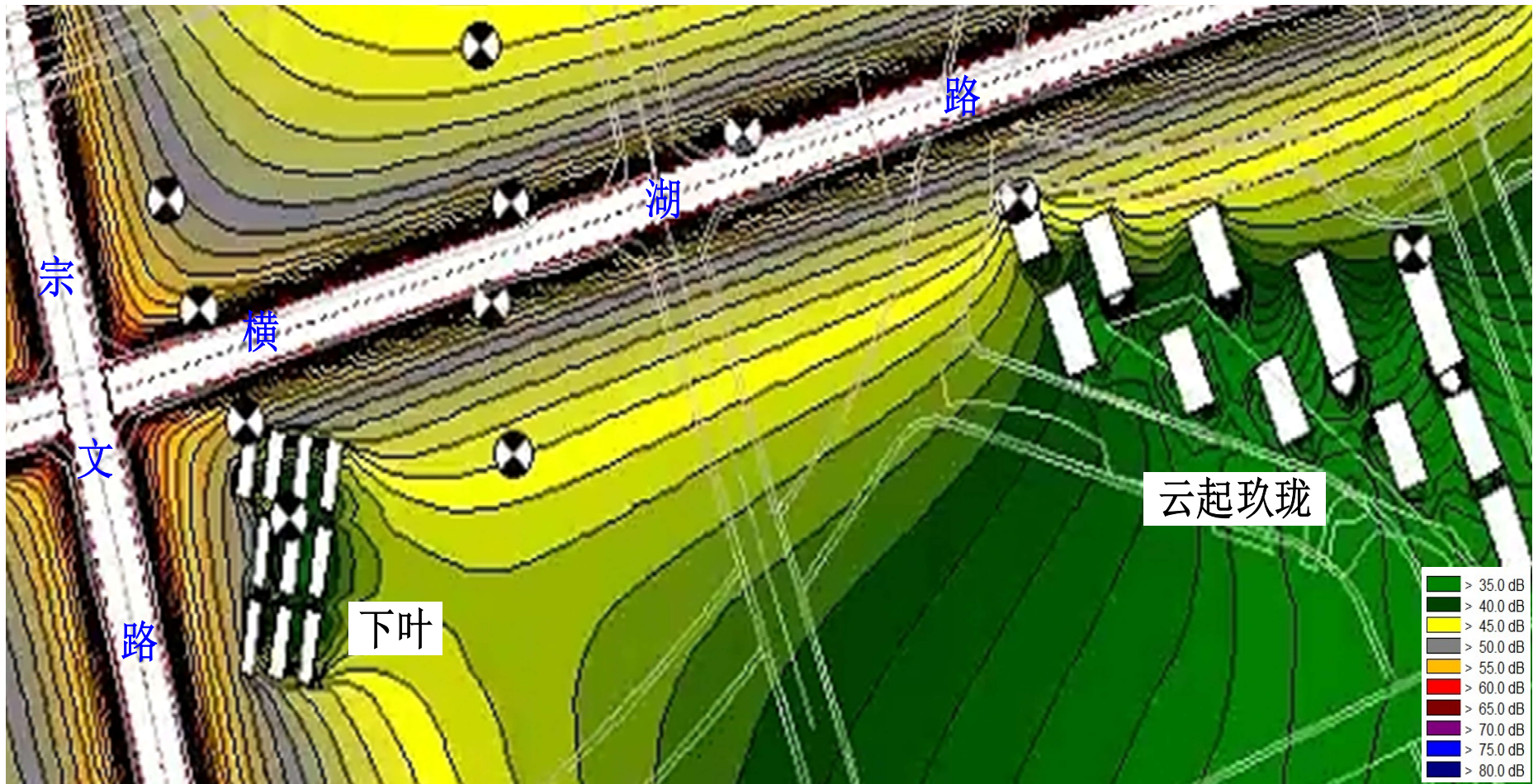
营运近期（2027年）夜间噪声等声级线图（本项目贡献值）
