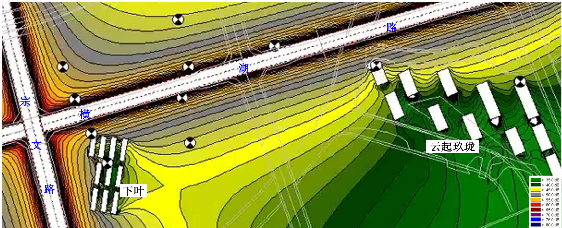
营运远期（2041年）夜间噪声等声级线图（本项目贡献值）
