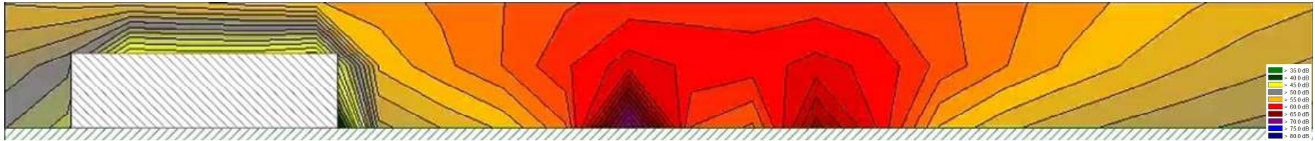
营运中期（2033 年）夜间下叶小区垂向噪声等声级线图
