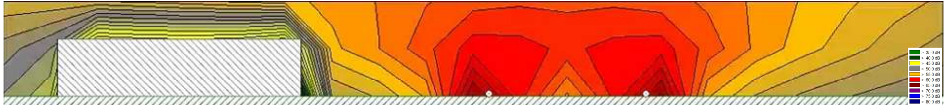
营运近期（2027年）夜间下叶小区垂向噪声等声级线图
