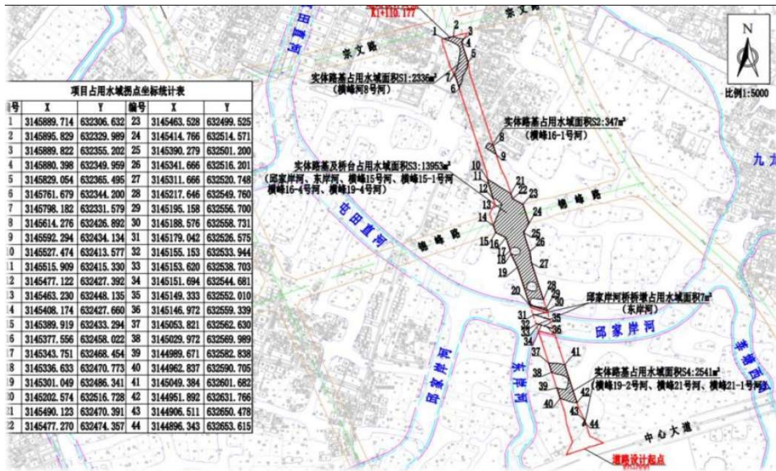
图 2-3 项目工程占用水域平面图
