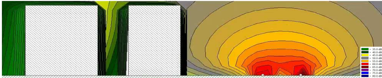
营运近期（2027年）夜间云起玖珑小区垂向噪声等声级线图
