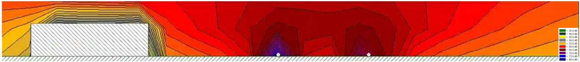
营运中期（2033 年）昼间下叶小区垂向噪声等声级线图
