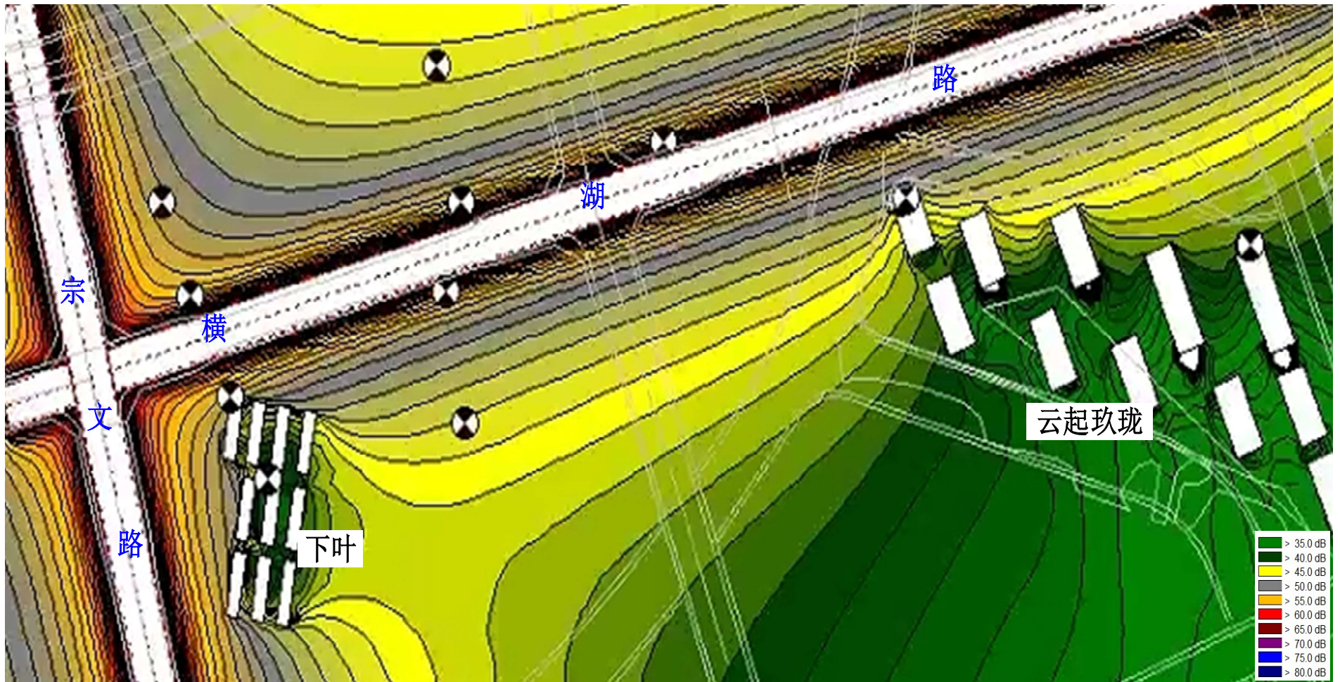
营运中期（2033年）夜间噪声等声级线图（本项目贡献值）
