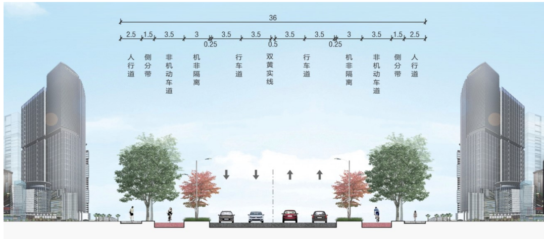
图 2-1 道路横断面布置图
