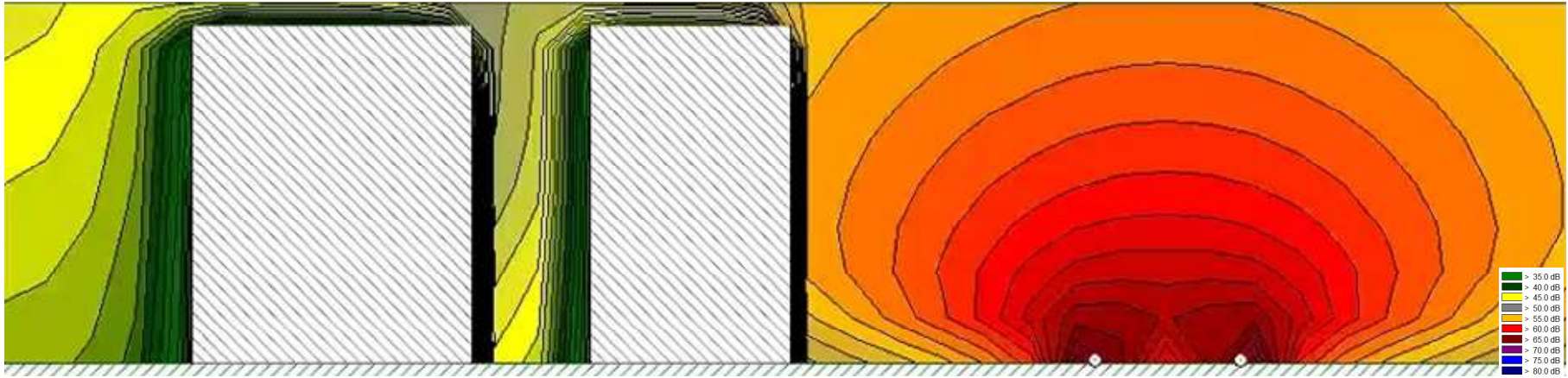
营运中期（2033年）昼间云起玫瑰小区垂向噪声等声级线图
