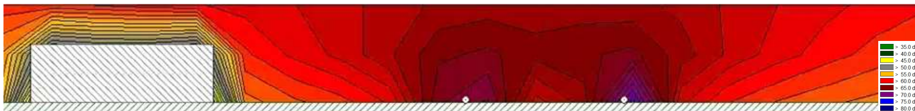
营运远期（2041 年）昼间下叶小区垂向噪声等声级线图
