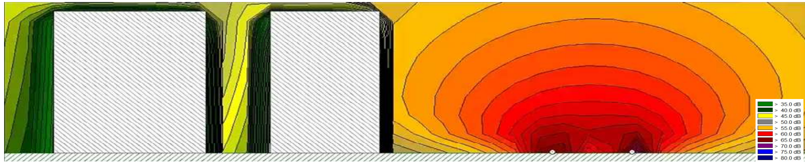
营运近期（2027年）昼间云起玖珑小区垂向噪声等声级线图
