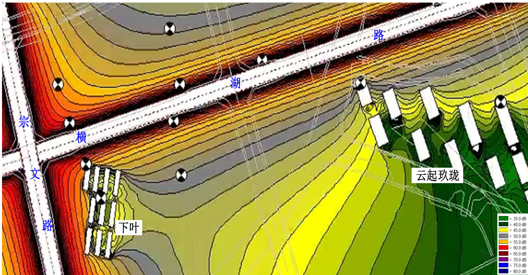
营运中期（2033年）昼间噪声等声级线图（本项目贡献值）
