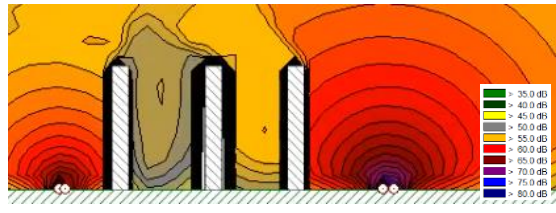
图 8-20 营运远期后洋吴苑昼间交通噪声立面等声级线图
