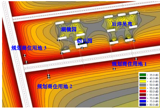
8-1 近期昼间交通噪声水平等声级线图
