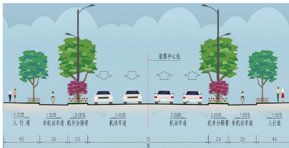
图 2-1 道路标准横断面
