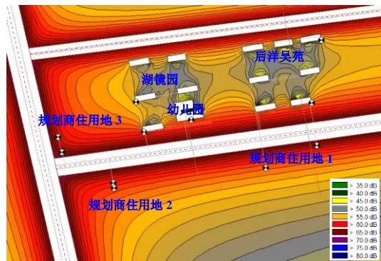
图 8-5 远期昼间交通噪声水平等声级线图
