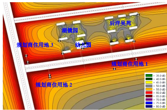
图 8-3 中期昼间交通噪声水平等声级线图
