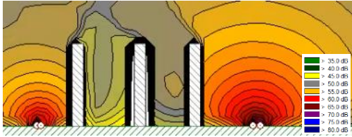
图 8-21 营运远期后洋吴苑夜间交通噪声立面等声级线图
