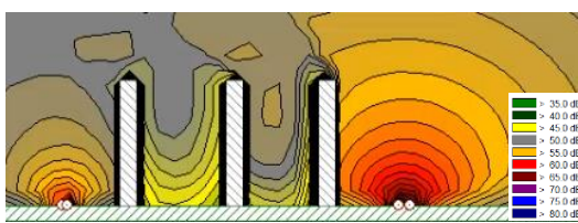
图 8-8 营运近期湖镜园夜间交通噪声立面等声级线图
