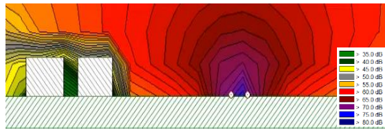
图 8-14 营运中期幼儿园昼间交通噪声立面等声级线图
