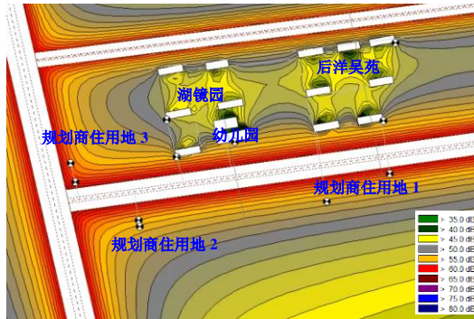
图 8-4 中期夜间交通噪声水平等声级线图
