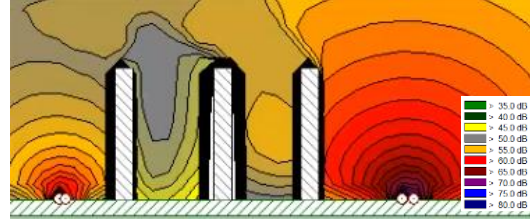
图 8-10 营运近期后洋吴苑昼间交通噪声立面等声级线图
