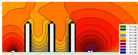
图 8-17 营运远期湖镜园昼间交通噪声立面等声级线图
