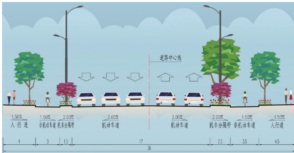
图 2-3 本项目道路与规划道路二交叉口渠化横断面图
