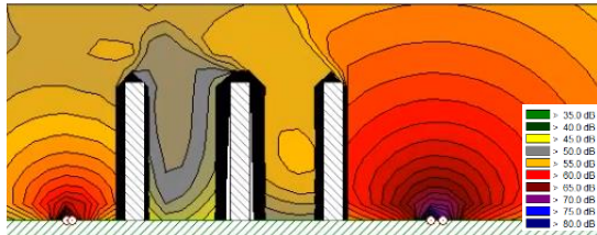
图 8-15 营运中期后洋吴苑昼间交通噪声立面等声级线图
