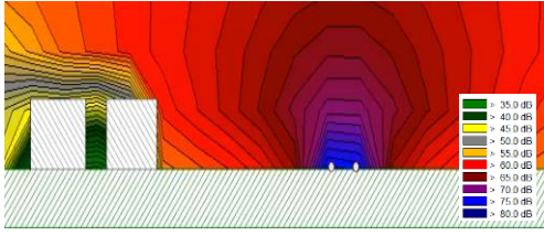
图 8-19 营运远期幼儿园昼间交通噪声立面等声级线图
