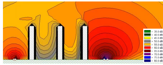
图 8-12 营运中期湖镜园昼间交通噪声立面等声级线图
