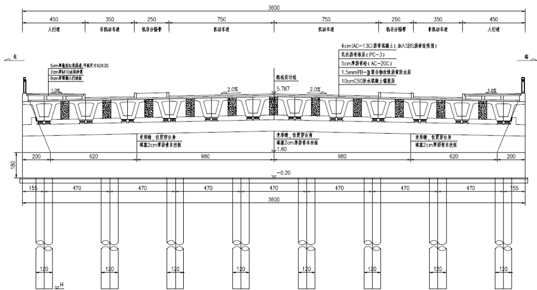
图 2-5 后洋河桥桥台正横断面布置图
