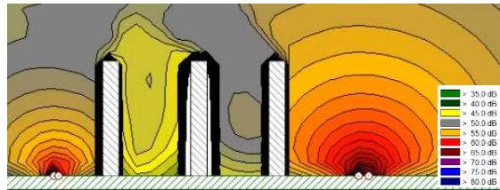
图 8-16 营运中期后洋吴苑夜间交通噪声立面等声级线图
