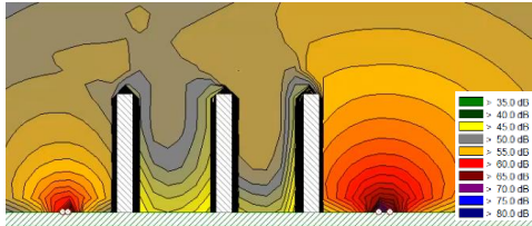
图 8-13 营运中期湖镜园夜间交通噪声立面等声级线图
