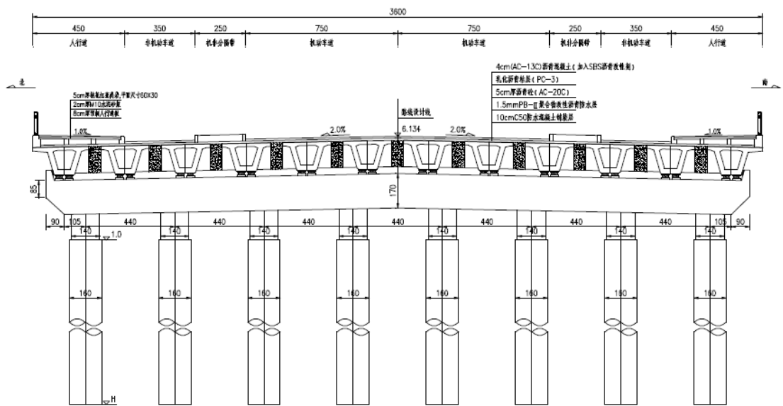
图 2-6 后洋河桥桥墩正横断面布置图
