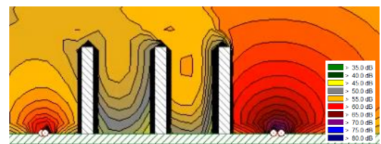
图 8-7 营运近期湖镜园昼间交通噪声立面等声级线图
