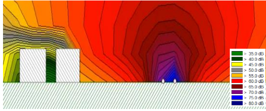
图 8-9 营运近期幼儿园昼间交通噪声立面等声级线图
