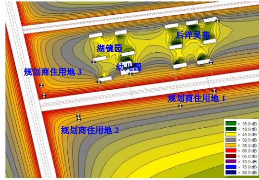
图 8-2 近期夜间交通噪声水平等声级线图
