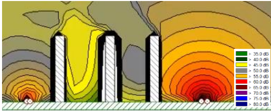
图 8-11 营运近期后洋吴苑夜间交通噪声立面等声级线图
