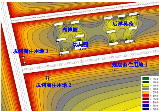
图 8-6 远期夜间交通噪声水平等声级线图
