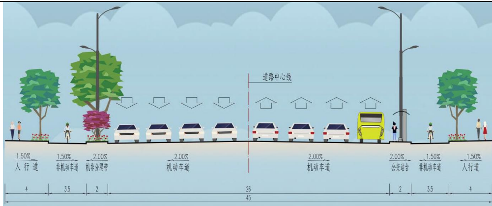
图 2-2 本项目道路与科创路交叉口渠化横断面图
